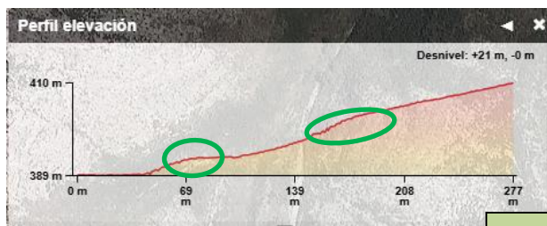
Perfil longitudinal del camino en todo uno. Con 2 zonas de pendientes del 12%-14%
