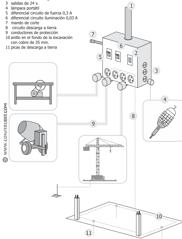
Instalación eléctrica. Esquema de instalación.
