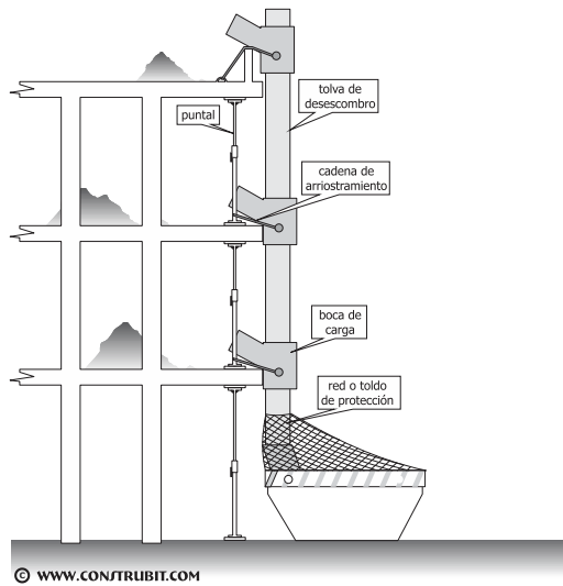
Tubo de desescombro. Vista lateral.
