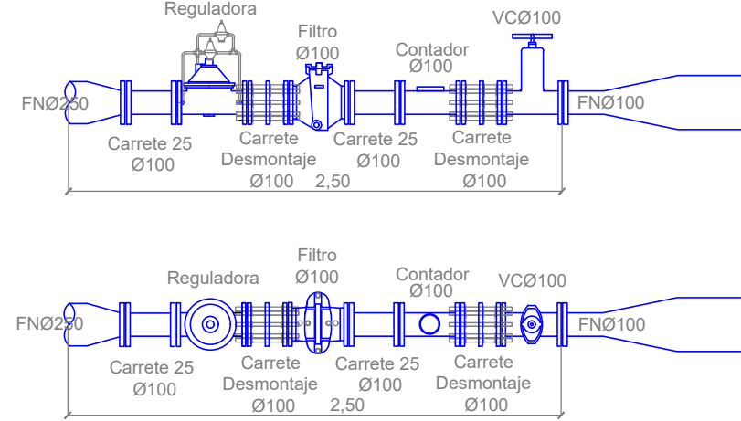
Regulación (Caudal) deposito PI
