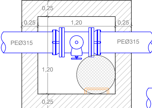
Arqueta Ventosa_Planta
