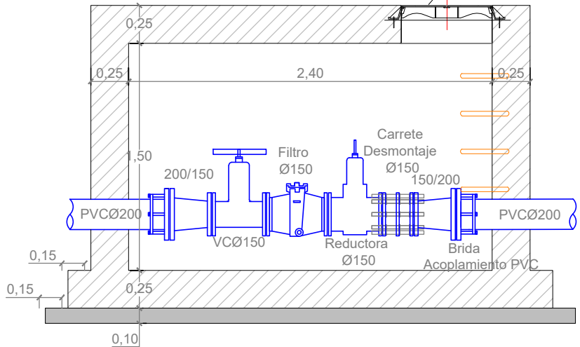
Regulación (presión) PB Iribas_Perfil
