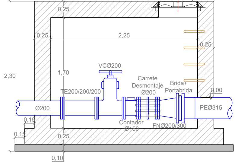
Nudo Manantial (NM)_Perfil
