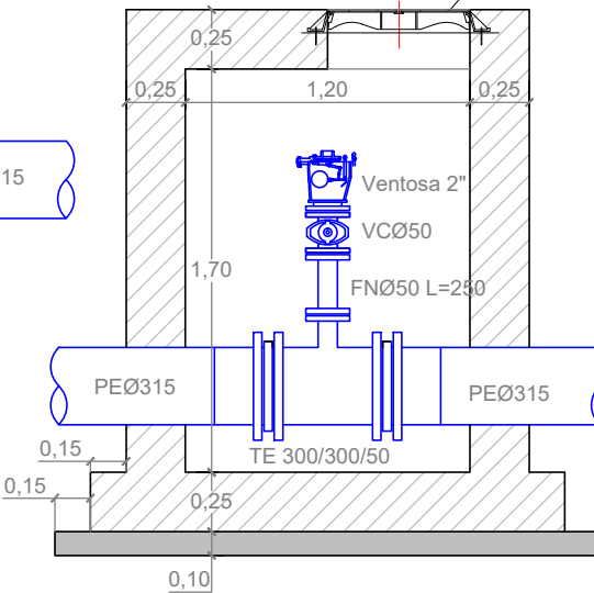
Arqueta Ventosa_Perfil
