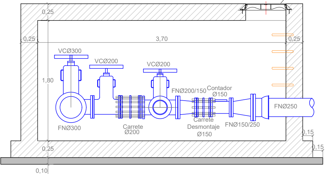
Regulación (Caudal) deposito PI
