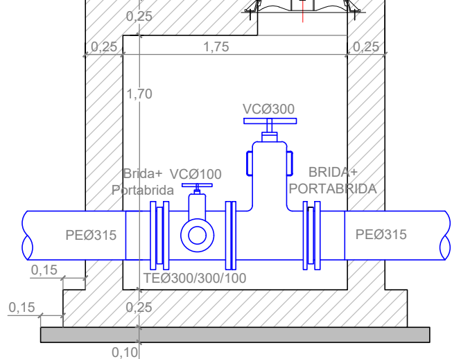
Arqueta Desagüe_Perfil
