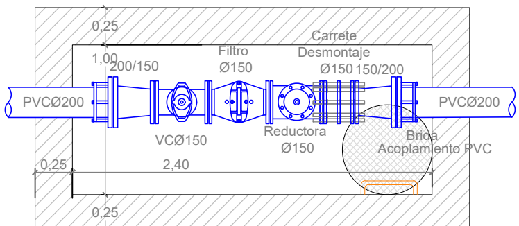
Regulación (presión) PB Iribas_Perfil
