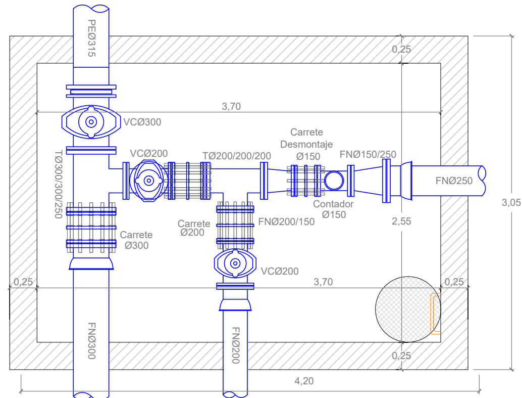
Nudo Ramal Poligono (NRPI)_Planta
