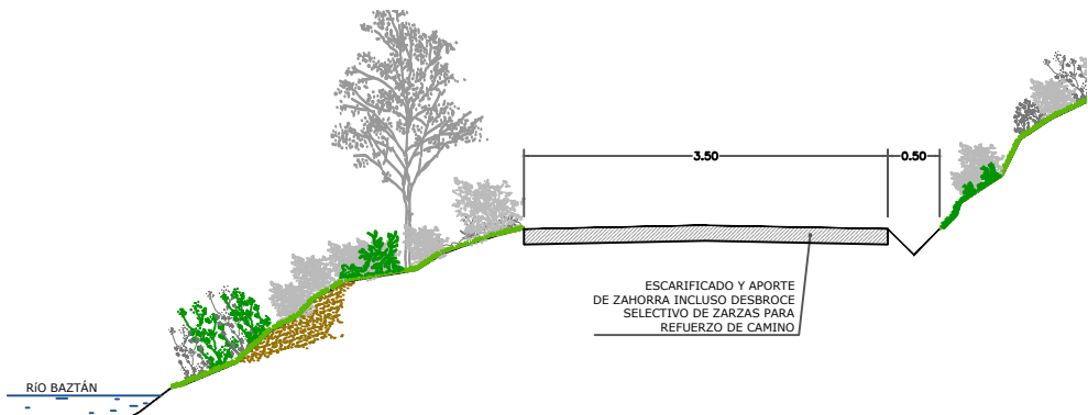
SECCIÓN TIPO H-H A1: 1/40 A3: 1/80
