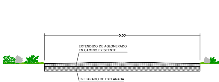
SECCIÓN TIPO D'-D' A1: 1/40 A3: 1/80
