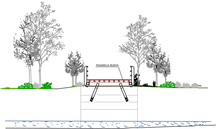
SECCIÓN TIPO Q-Q A1: 1/40 A3: 1/80
