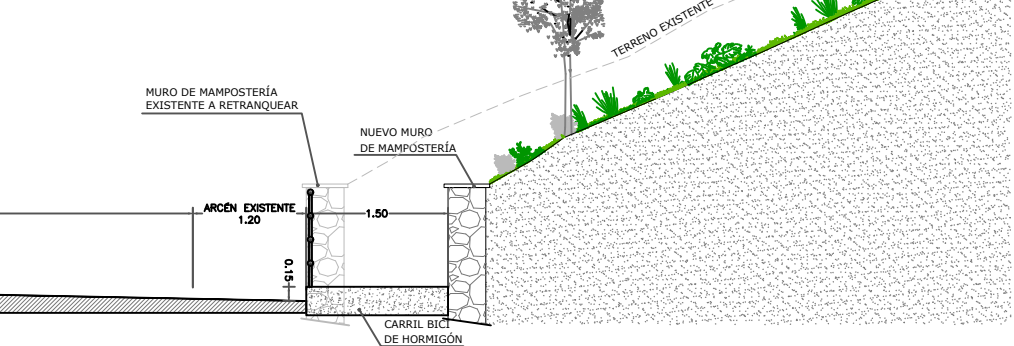
SECCIÓN TIPO F-F A1: 1/40 A3: 1/80
