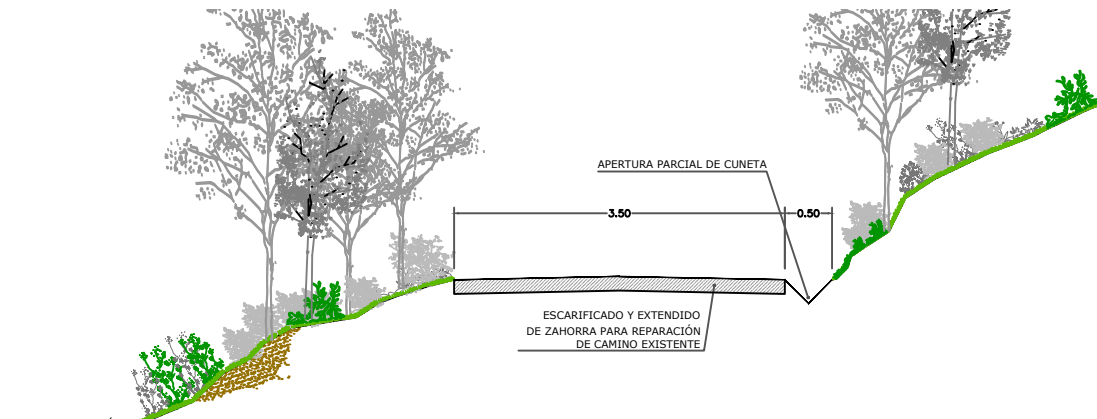
SECCIÓN TIPO O-O A1: 1/40 A3: 1/80
