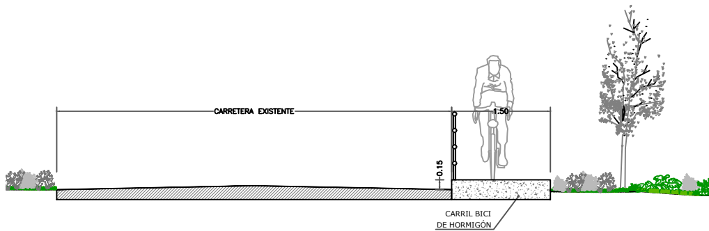
SECCIÓN TIPO C'-C' A1: 1/40 A3: 1/80
