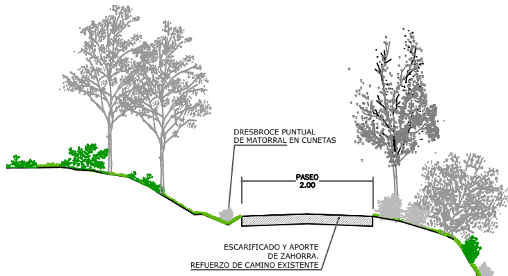
SECCIÓN TIPO D'-D' A1: 1/40 A3: 1/80
