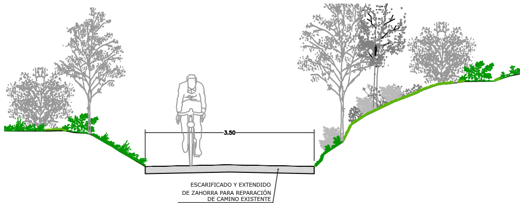
SECCIÓN TIPO C-C A1: 1/40 A3: 1/80
