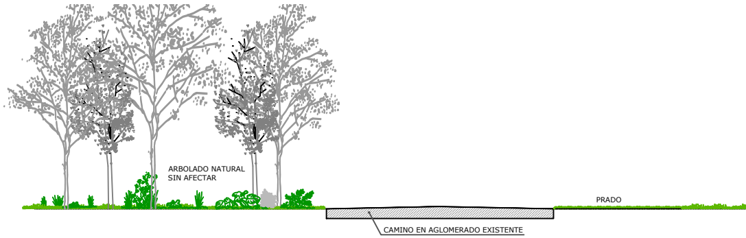
SECCIÓN TIPO R-R A1: 1/40 A3: 1/80
