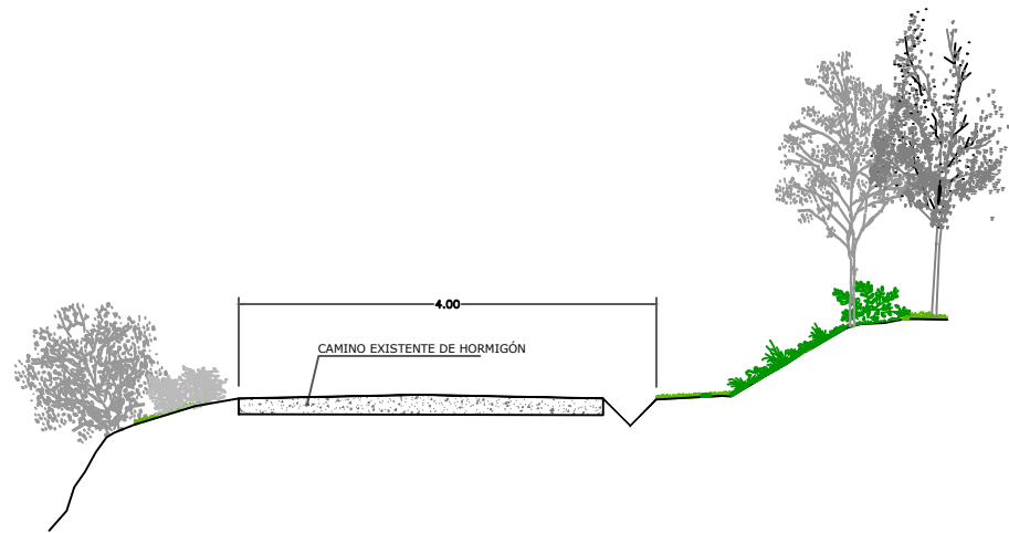
SECCIÓN TIPO B-B A1: 1/40 A3: 1/80
