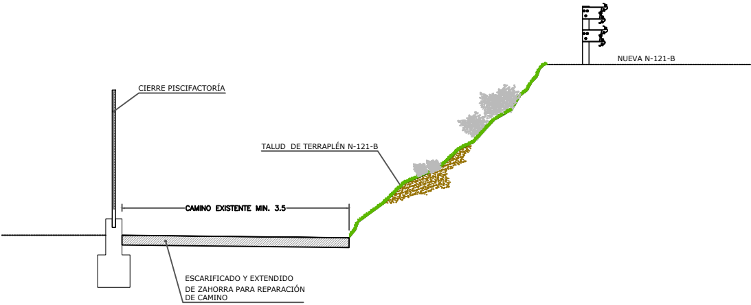
SECCIÓN TIPO N-N A1: 1/40 A3: 1/80
