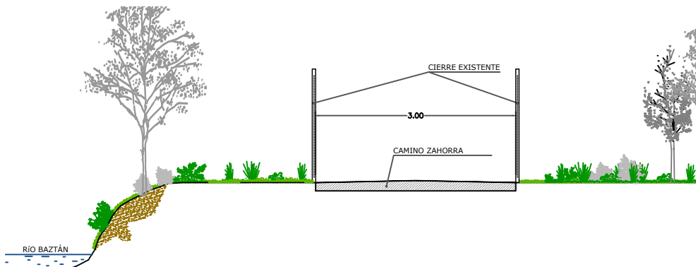
SECCIÓN TIPO L-L A1: 1/40 A3: 1/80
