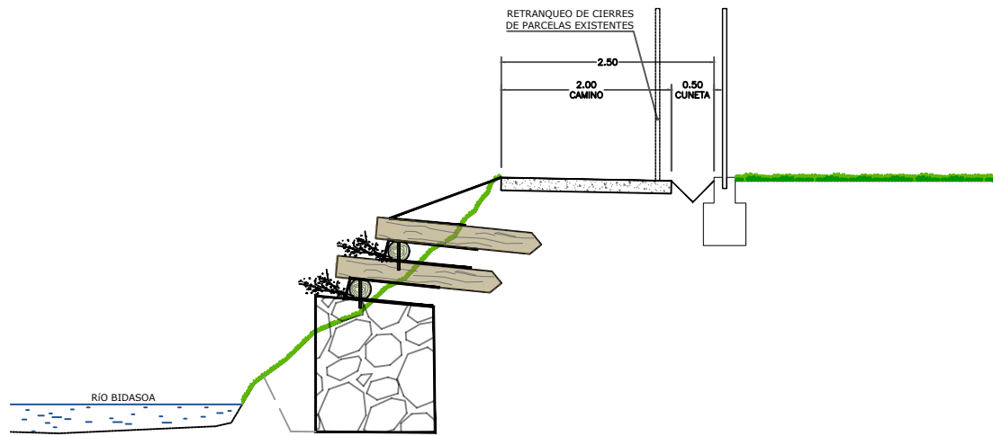
SECCIÓN TIPO A-A A1: 1/40 A3: 1/80
