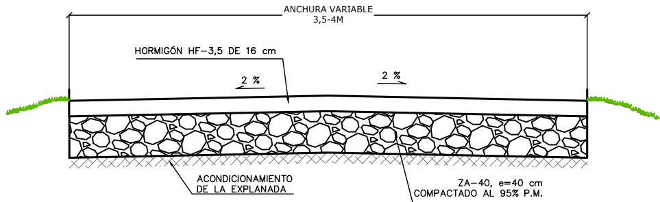
SECCIÓN TIPO CAMINO NUEVO DE HORMIGÓN
