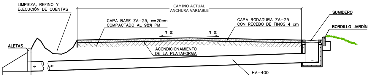
SECCIÓN TIPO CON CRUCE DE CUNETAS
