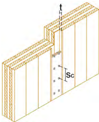
Figura: Junta en paneles verticales – Junta con tabla lateral de madera (tabla a tope)
