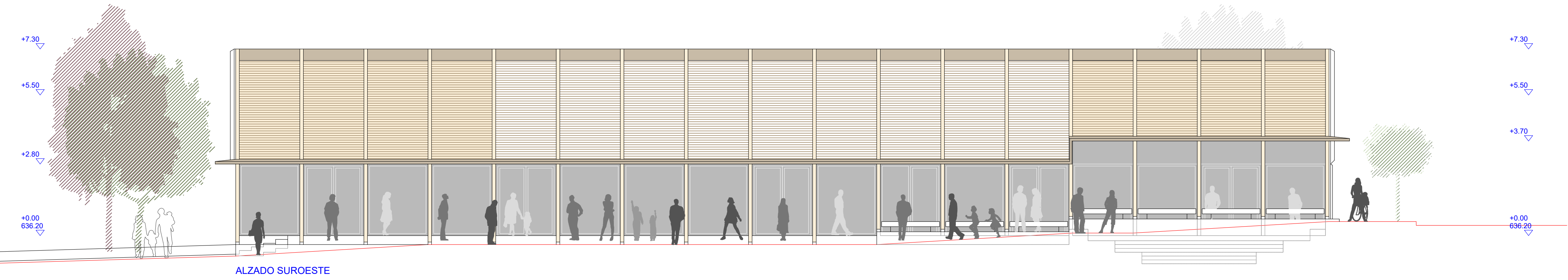
ALZADO SUROESTE
