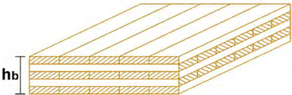
Figura: Características geométricas de forjado CLT
