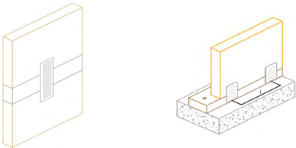
Figura: representación gráfica de conexión madera a madera con placas perforadas de metal.
