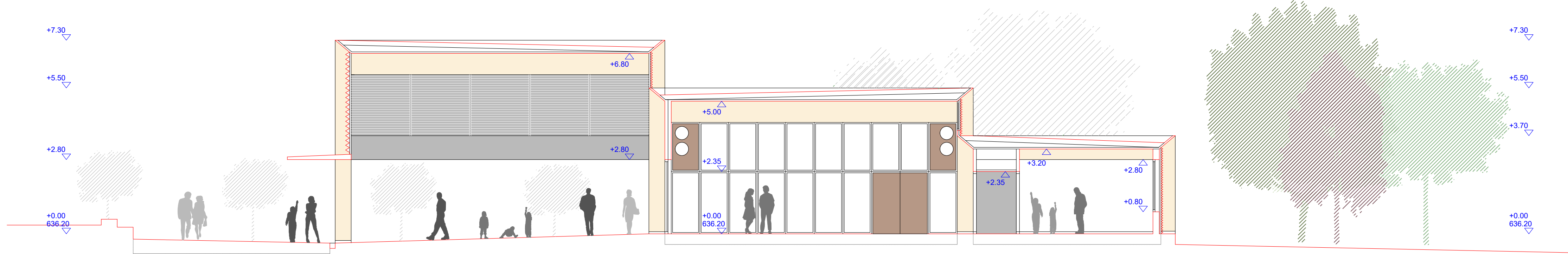
SECCIÓN TRANSVERSAL I
