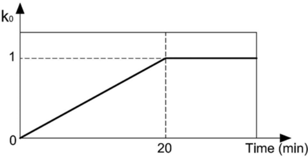
Figure: Variación de k_0 para elementos sin protección.
