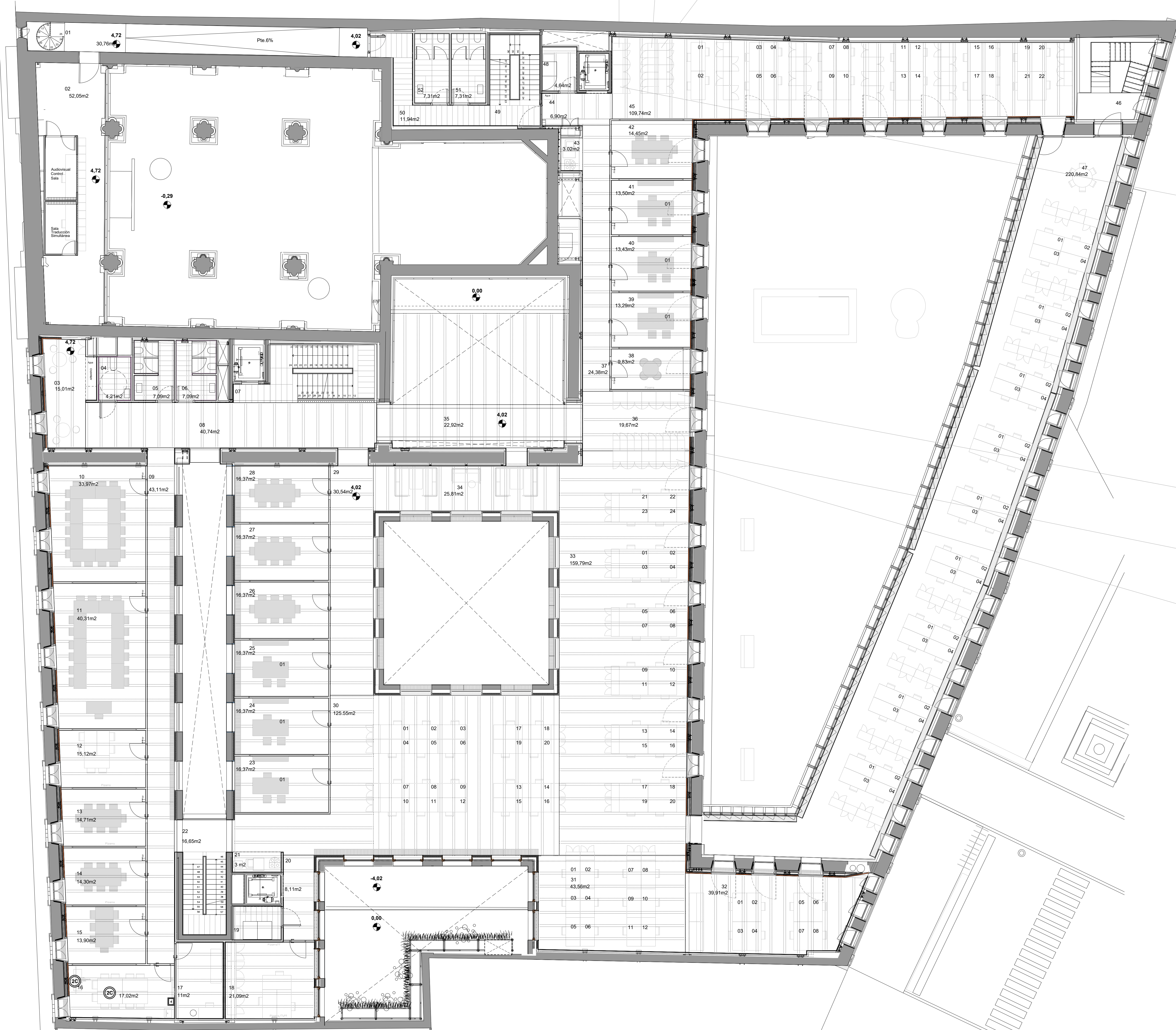
ARMARIOS PLANTA 1
