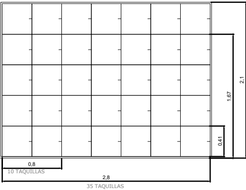
1 LÍNEAS DE TAQUILLAS
