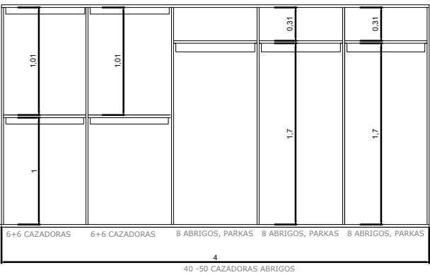
INTERIOR - 2 barras de colgar
