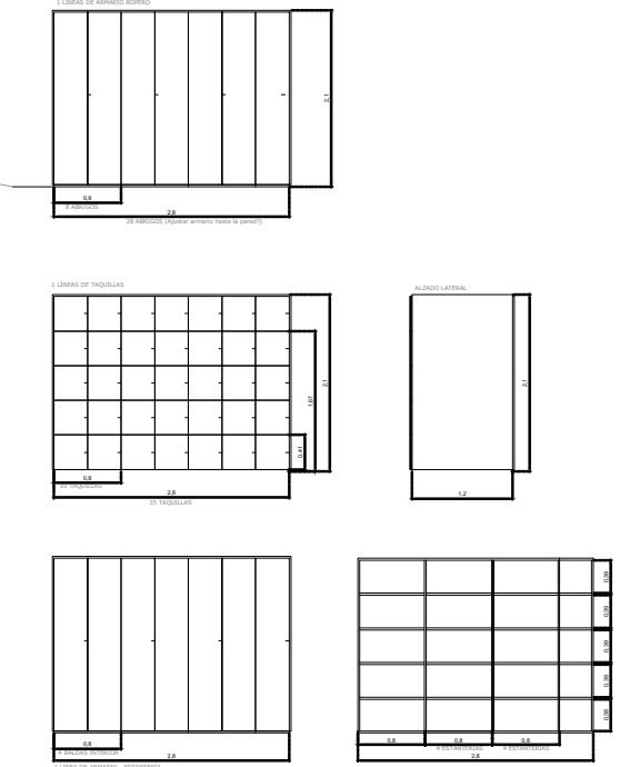
ARMARIOS PLANTA 1
