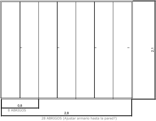
1 LÍNEAS DE ARMARIO ROPERO
