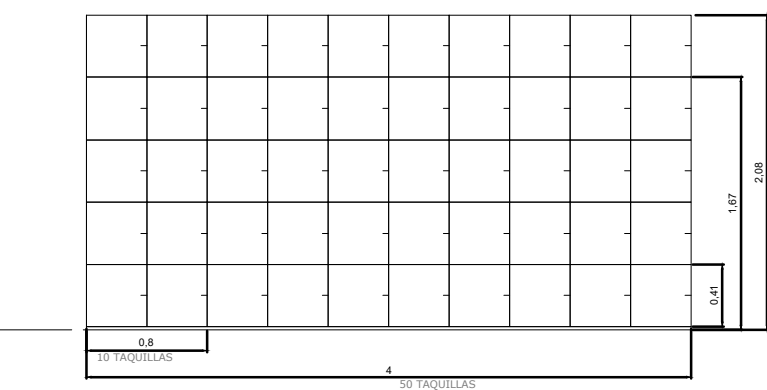
1 LÍNEAS DE TAQUILLAS
