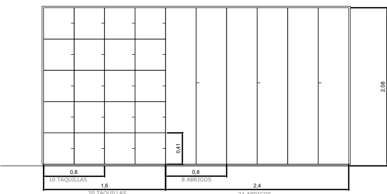
1 LÍNEA DE TAQUILLAS + ARMARIOS ROPEROS - BALDAS
