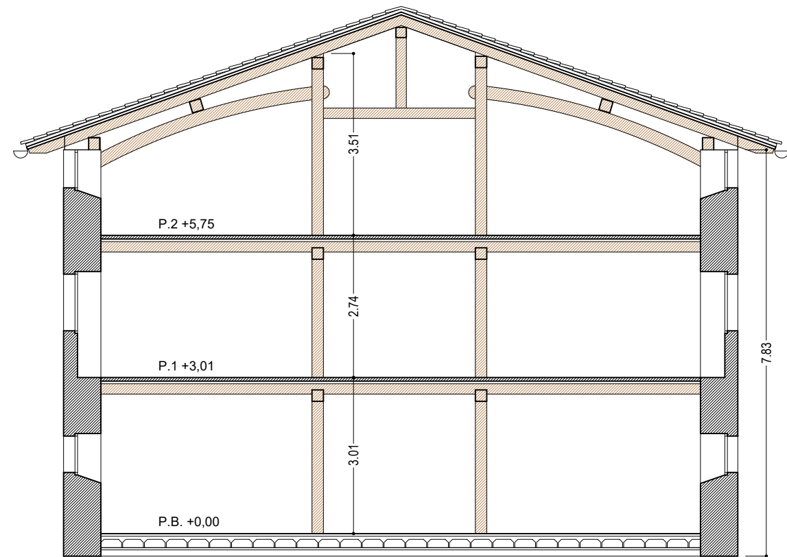
SECCIÓN
