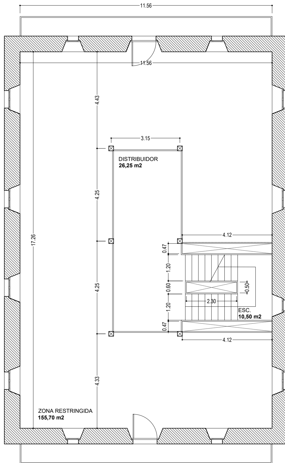
PLANTA SEGUNDA
