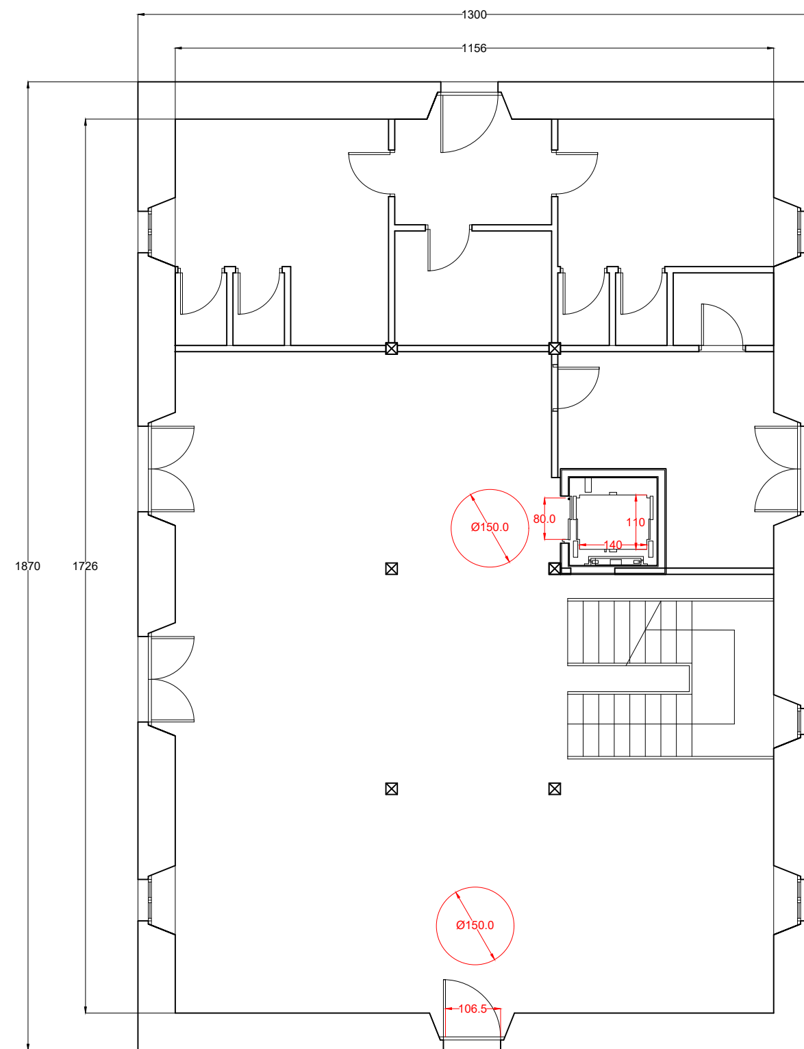
PLANTA BAJA
