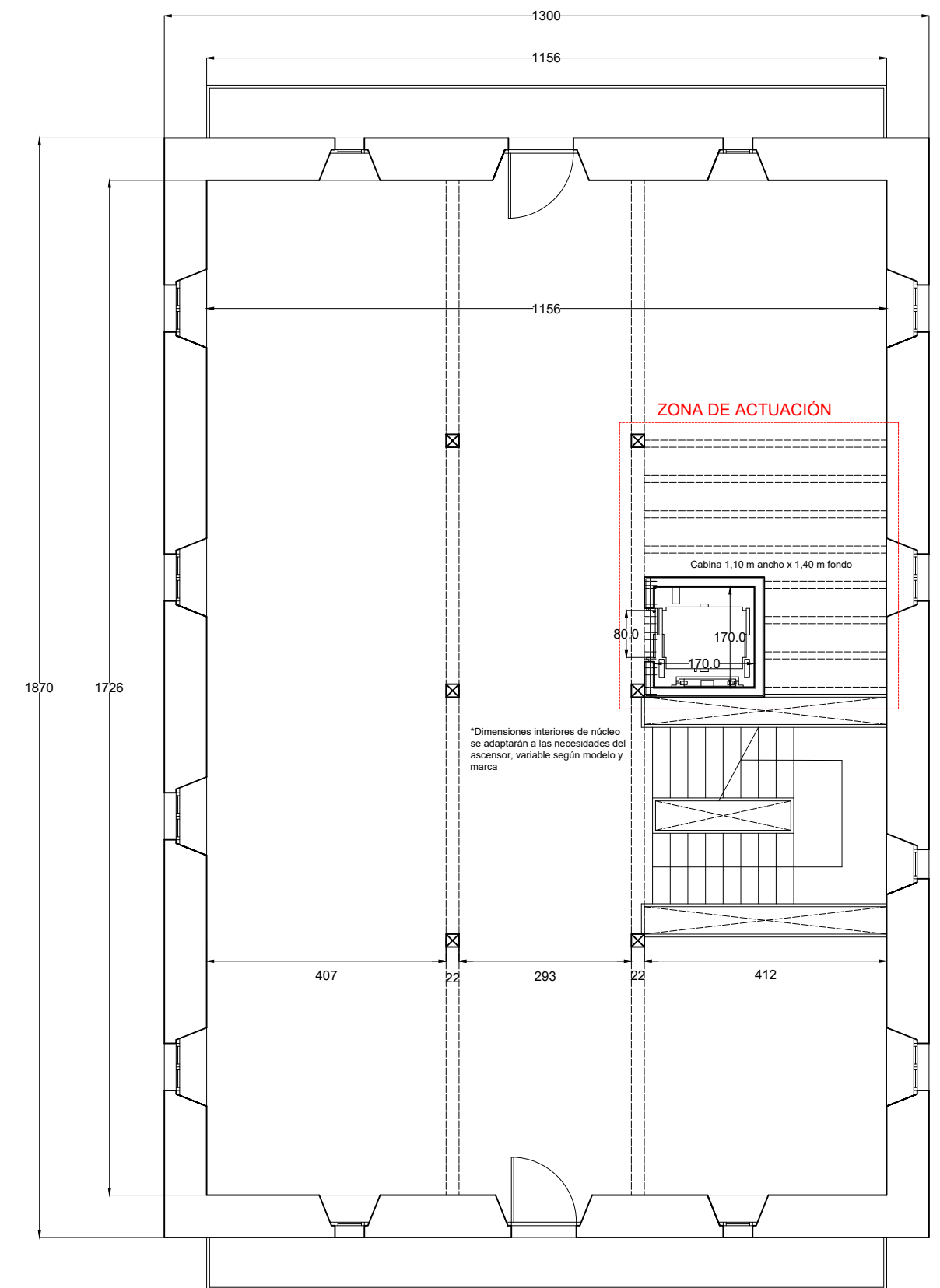
PLANTA SEGUNDA
