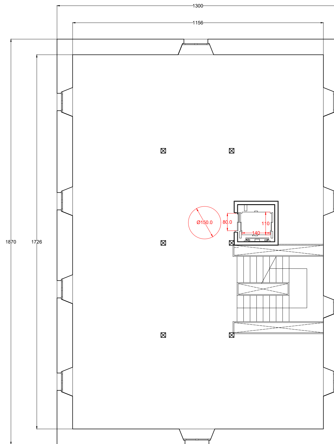
PLANTA PRIMERA
