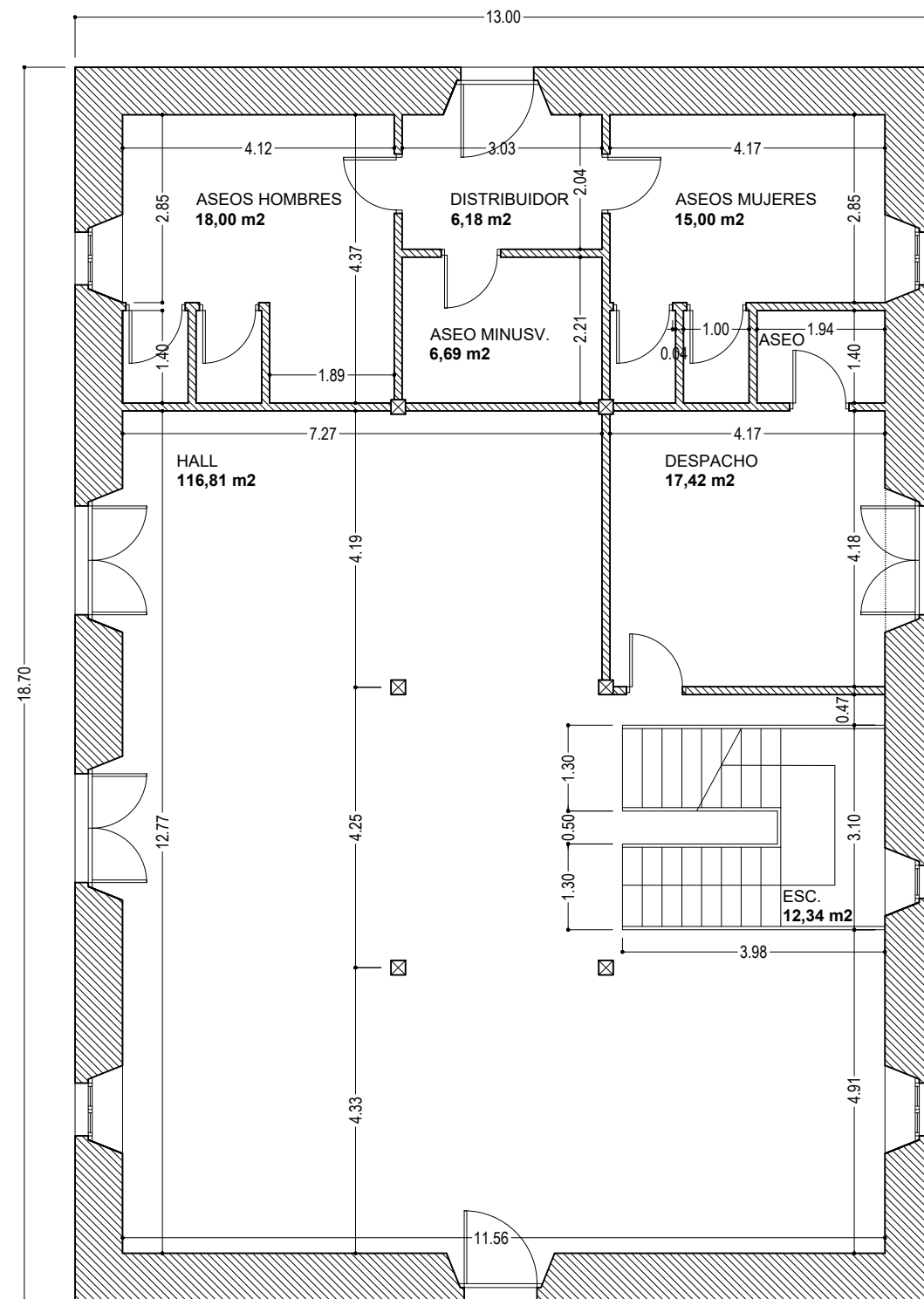
PLANTA BAJA
