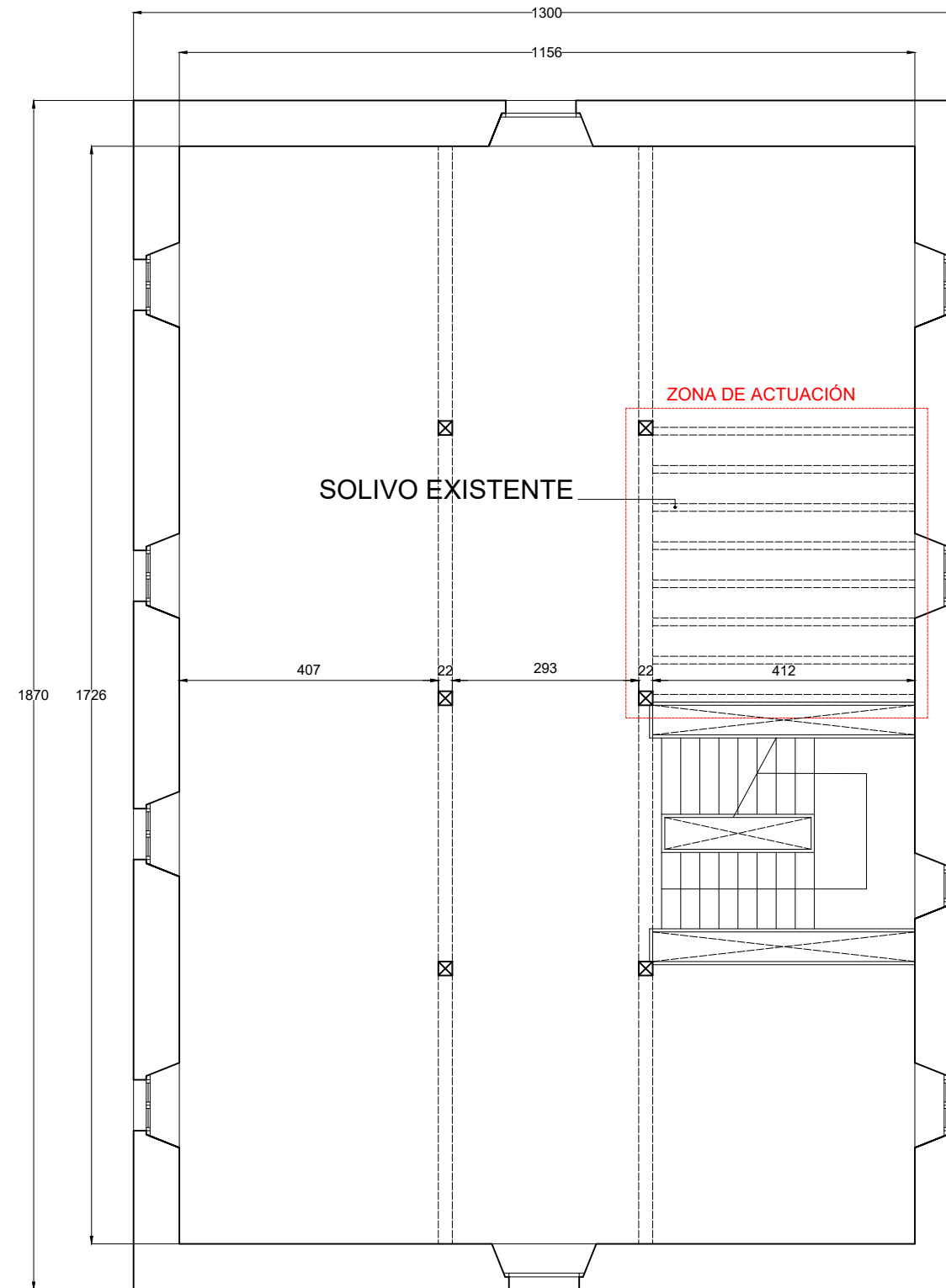
PLANTA PRIMERA
