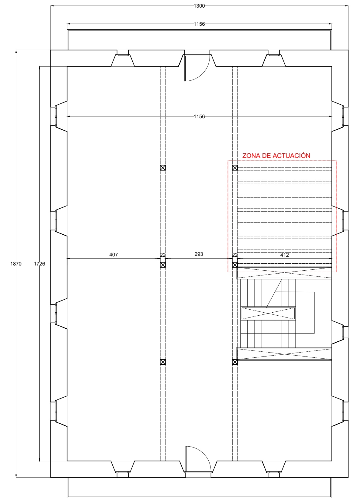
PLANTA SEGUNDA
