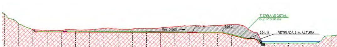
Secciones tipo inicial y final de la plataforma de la zona B
