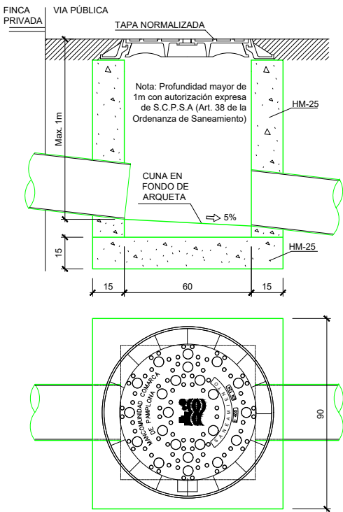
ARQUETA ACOMETIDA H>70 CM E=1/25
