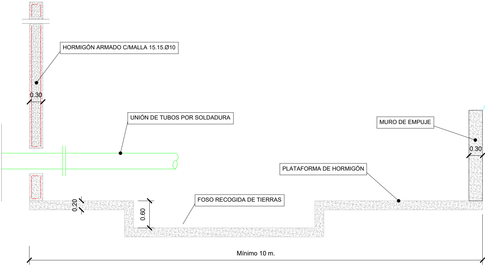
SECCIÓN LONGITUDINAL
