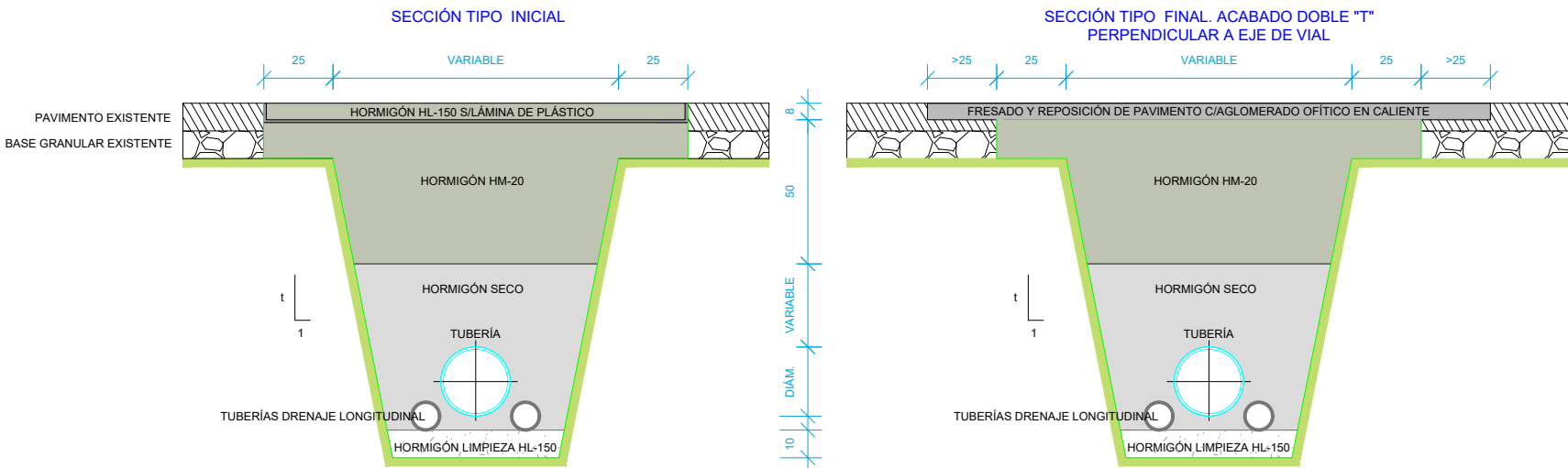
ZANJA EN CRUCE DE CARRETERAS Y CAMINOS. E=1/25
