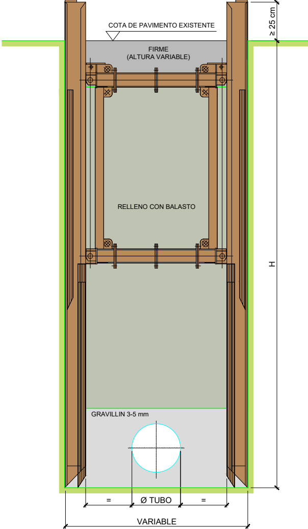
ZANJA TIPO ENTIBADA. E=1/25
