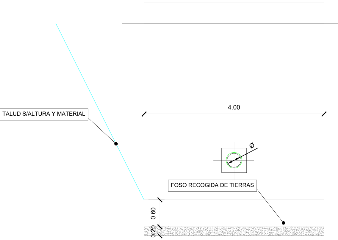
SECCIÓN TRANSVERSAL
