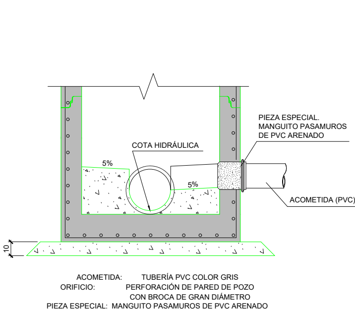
INCORPORACIÓN DE ACOMETIDA A POZO E=1/25
