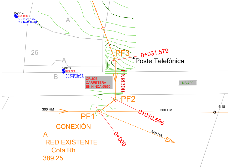
SITUACIÓN PERFORACIÓN EN HINCA E: 1/1000
