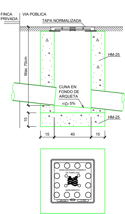
ARQUETA ACOMETIDA H<70 CM E=1/25
