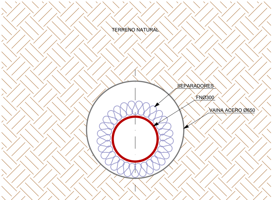
DETALLE PERFORACIÓN EN HINCA E: 1/1000
