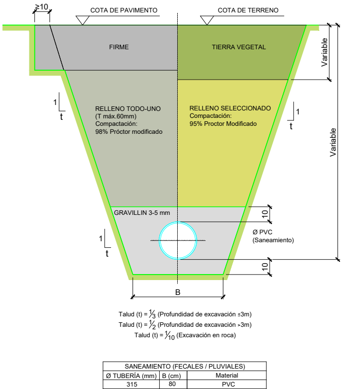
ZANJA TIPO SANEAMIENTO PVC. E=1/25
