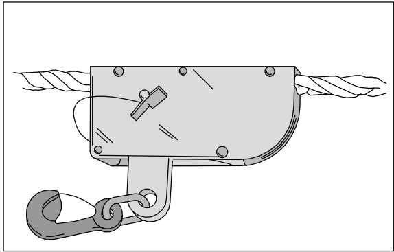
Andale móvil para cinturón de seguridad
