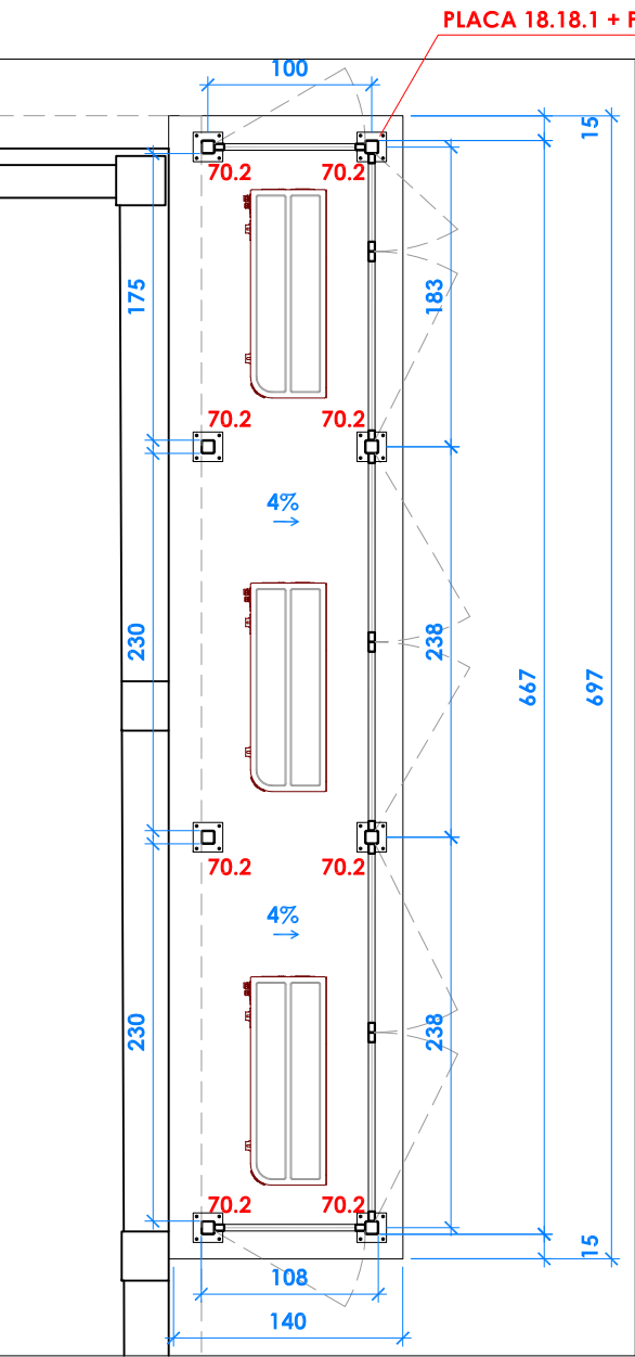
PLANTA COTA 0
