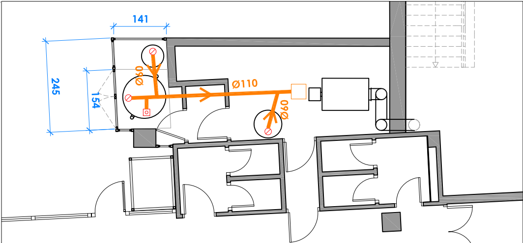
SALA DE CALDERAS. PLANTA SEMISÓTANO
