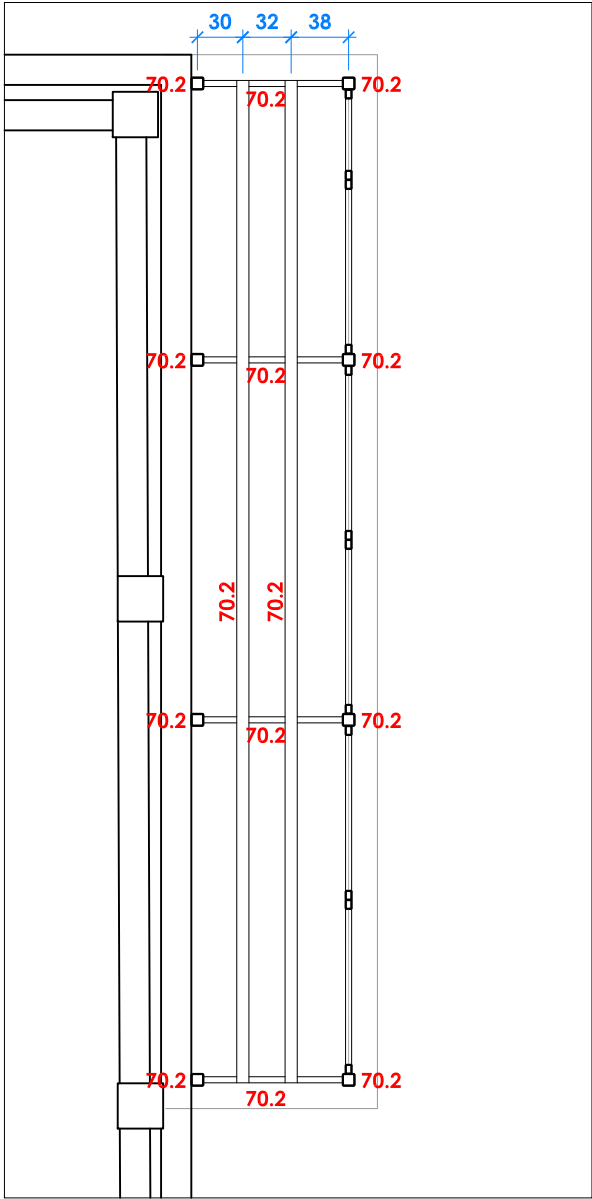
PLANTA INTERMEDIA
