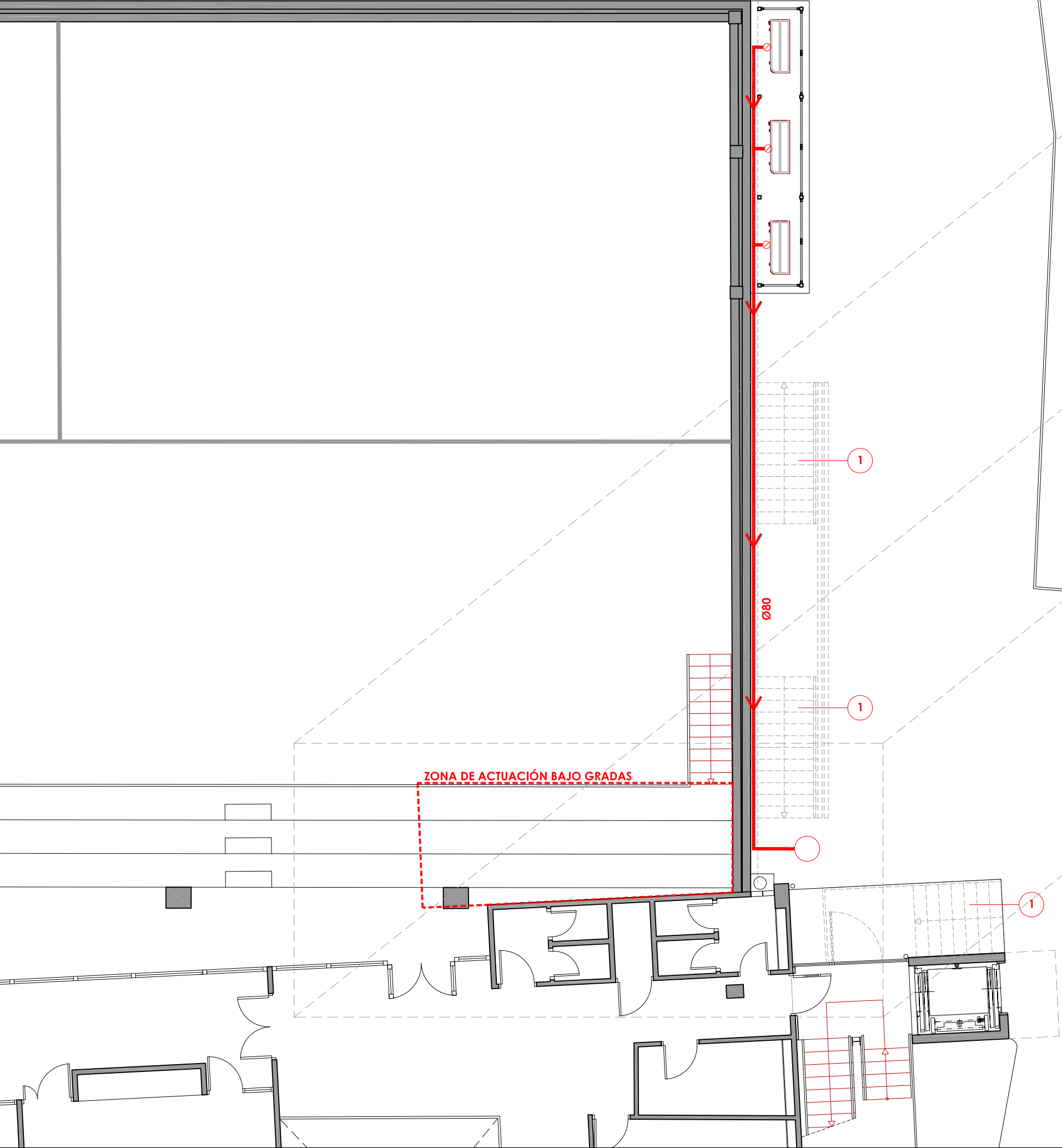
SALA DE CALDERAS. PLANTA SEMISÓTANO
