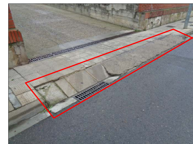
⑬ DEMOLICIÓN VADO Y DESPLAZAMIENTO DE SUMIDERO EN ACCESO APARCAMIENTO PISCINAS
