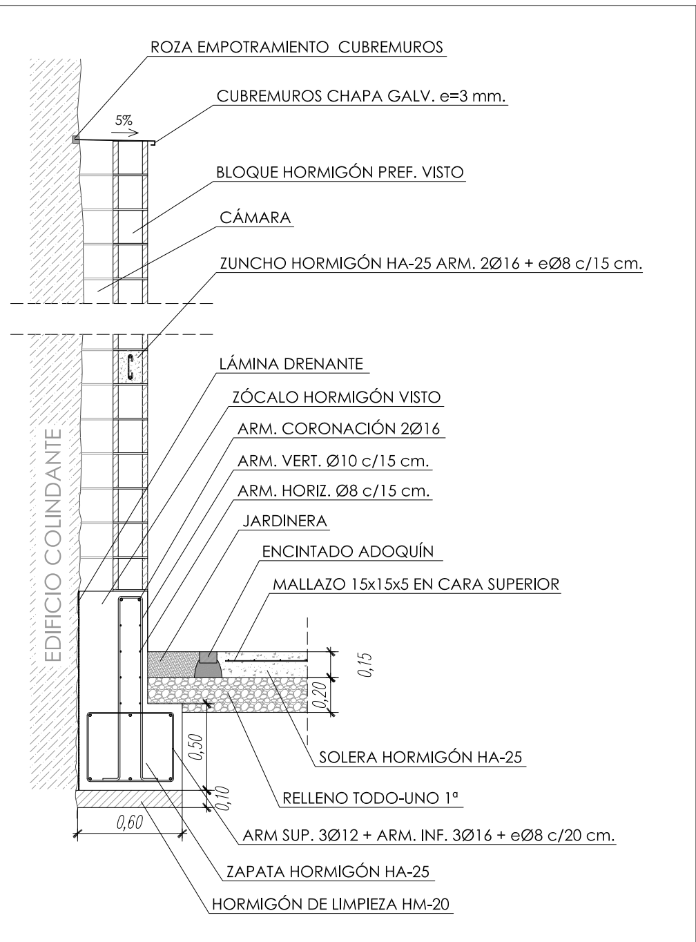
SECCIÓN CERRAMIENTO
