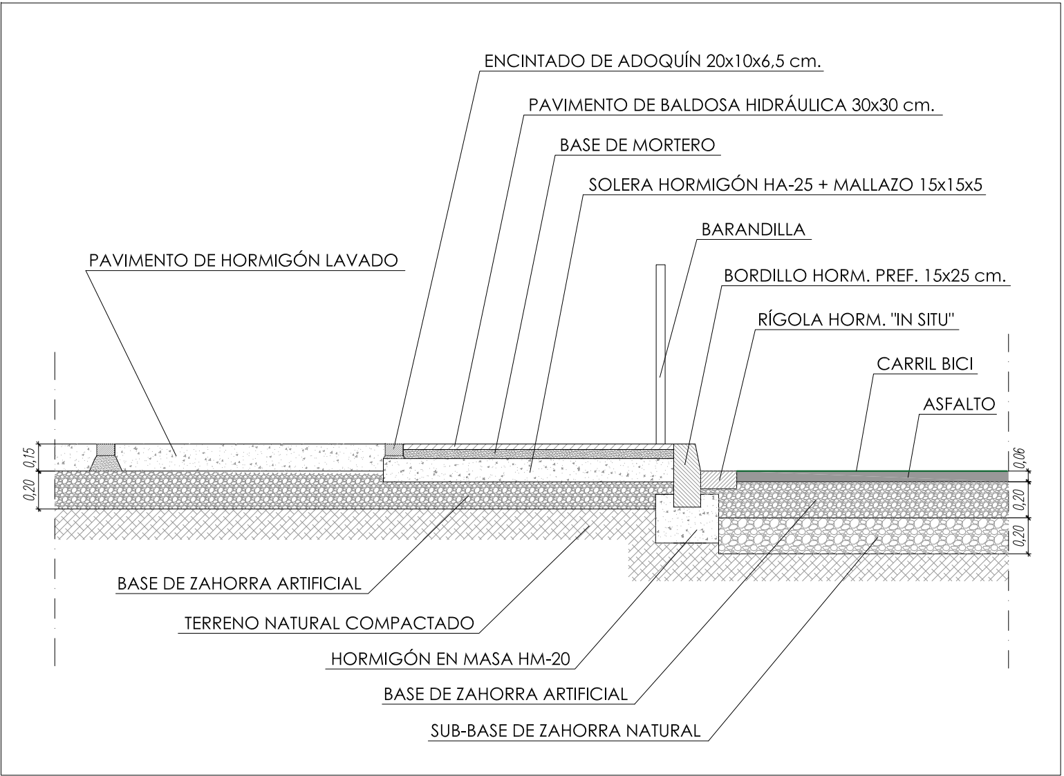
SECCIÓN A-A'
