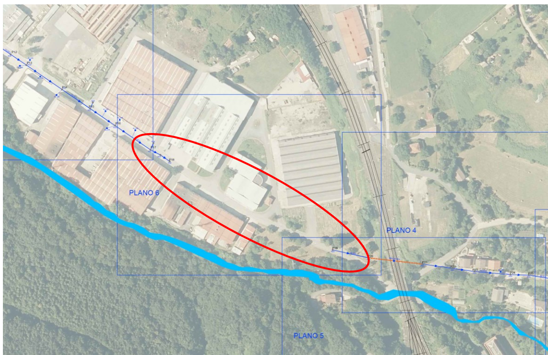
Plano de la situación de los colectores de saneamiento en el polígono industrial Ibarrea. Se señala en rojo el tramo que se encuentra sin renovar, y sobre los que se plantea intervenir.
