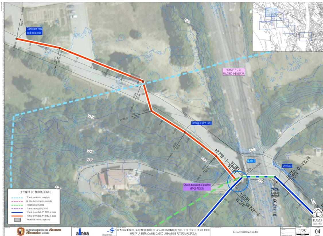
Detalle de la actuación realizada de abastecimiento hasta el inicio del polígono industrial Ibarrea.
