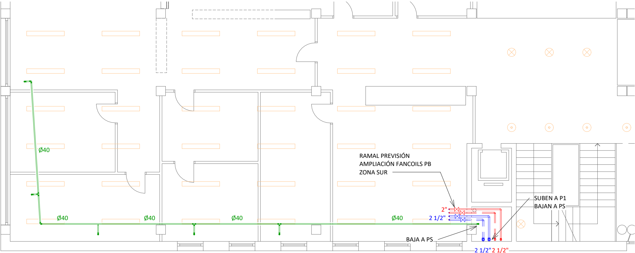
2 PLANTA BAJA 1 : 100
