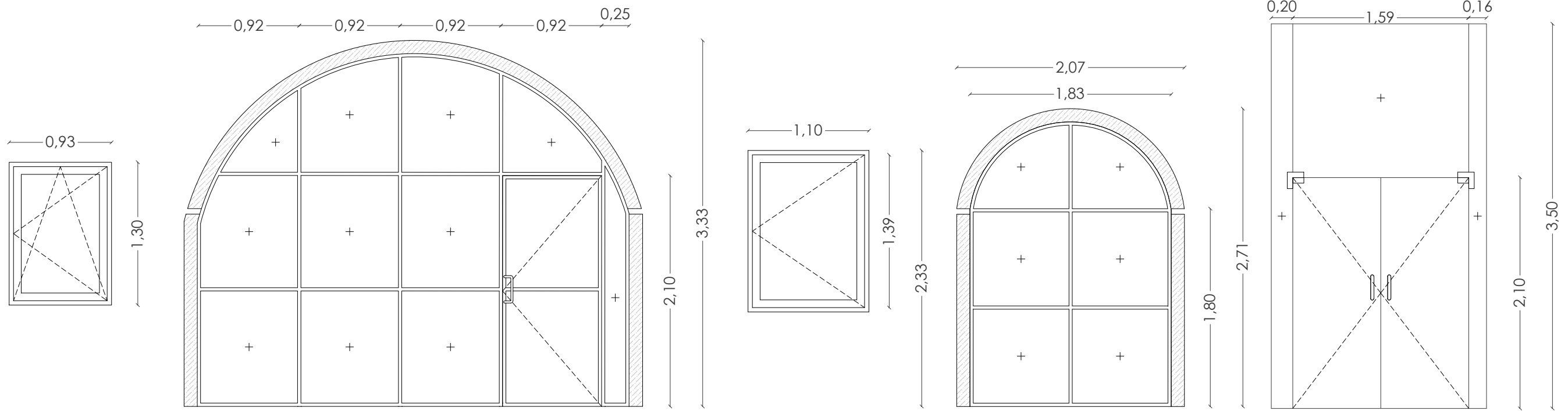
V5 1 hoja oscilo batiente. 1 unidad. Planta primera. Carpintería acero RPT. V6 11 hojas fijas.1 hoja abatible. 1 unidad. Planta baja. Carpintería acero. 4 Pernios antipalanca de acero inox mate y cerradura V1 1 hoja abatible. 1 unidad. Planta baja Carpintería de acero V2 6 hojas fijas. 1 unidad. Planta baja Carpintería de acero. V7 3 hojas fijas.2 hojas abatible. 1 unidad. Planta segunda. Herrajes de acero.
