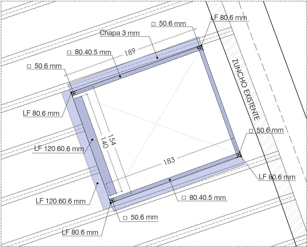
TECHO PLANTA BAJA
