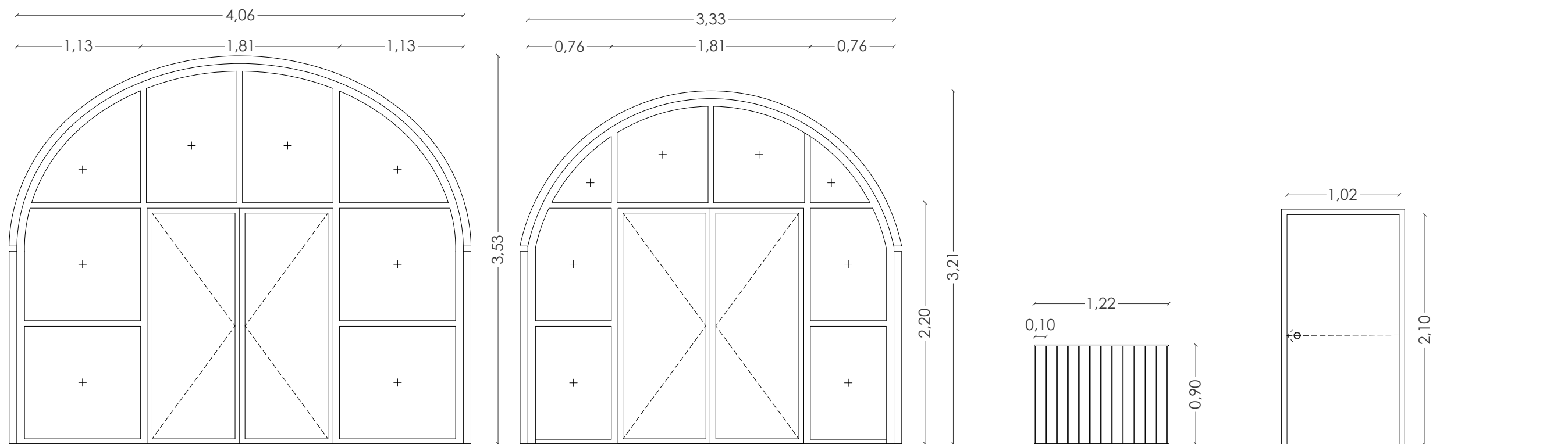
V3 8 hojas fijas. 2 hojas abatibles 1 unidad. Planta baja Carpintería de acero RPT. V4 8 hojas fijas. 2 hojas abatibles 1 unidad. Planta baja Carpintería de acero RPT. B1 Barandilla altura 90 cm Barroteado Ø8 mm P1 1 hoja corredera. Guia interior. 3 unidades. Planta baja y primera. Carpintería de DM 3 pernios de acero inoxidable mate. Manilla de acero inoxidable mate a ambos lados. Condena operable desde el exterior en baños.
