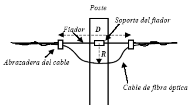
Figura 10 Fijación del cable.
