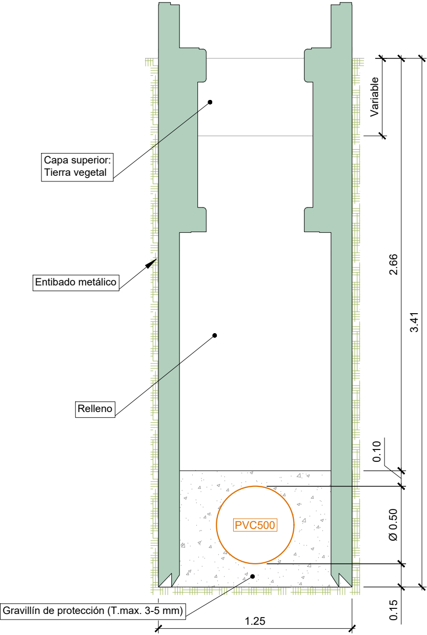
SECCIÓN TIPO ZANJA ENTIBADA PARA TUBERÍA PVC500 E=1/25
