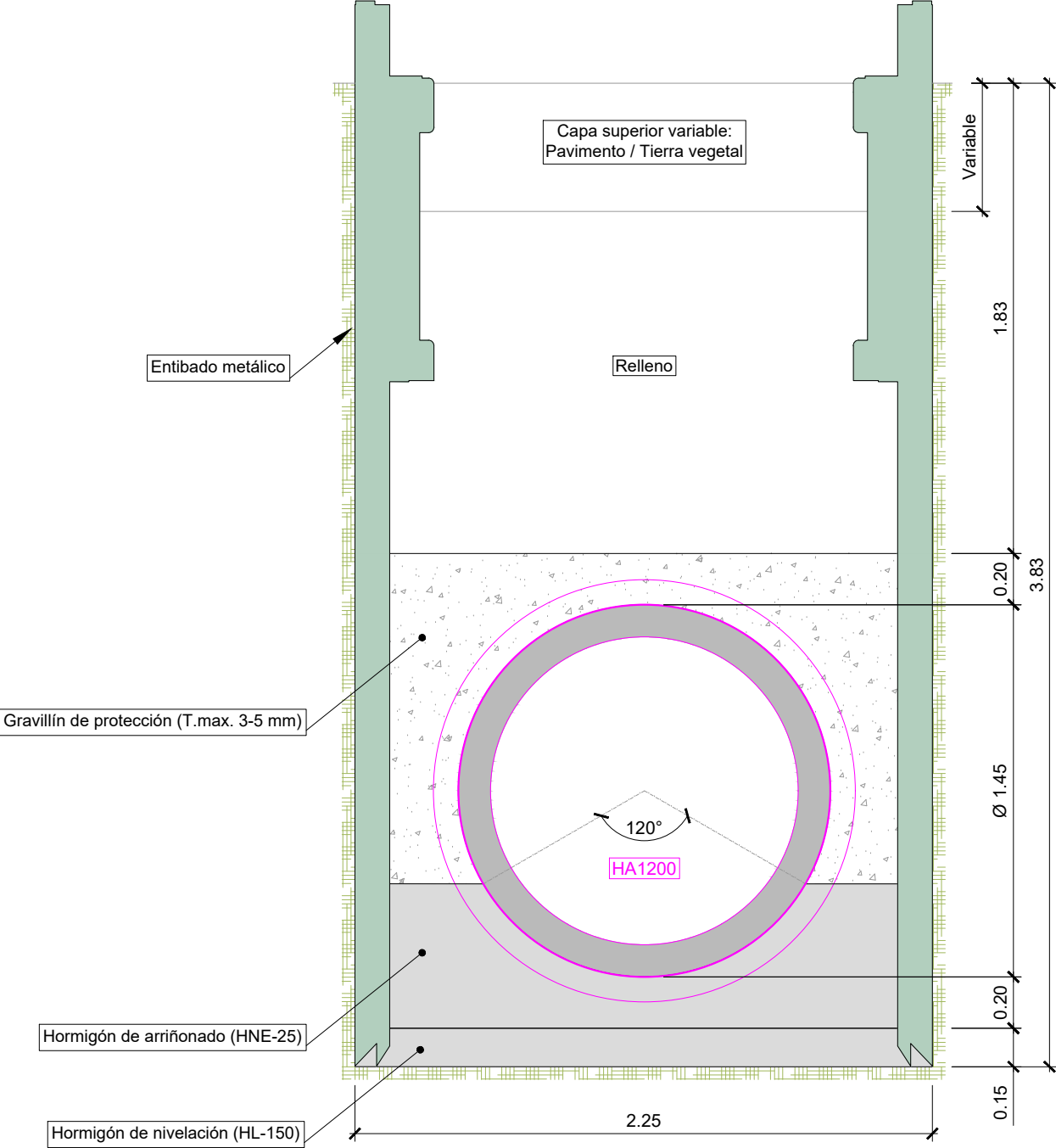
SECCIÓN TIPO ZANJA ENTIBADA PARA TUBERÍA HA1200 E=1/25
