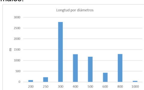
Longitudes por dimensión máxima
