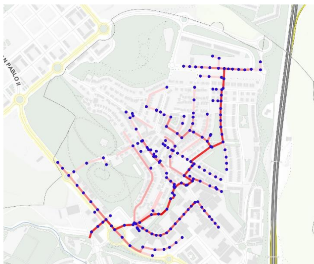
Red de Pluviales analizada: se representan los colectores en tonos de rojo. En oscuro los de mayor diámetro (DN800) y más claros a medida que disminuye el diámetro. En azul, quedan representados los pozos de registro.
