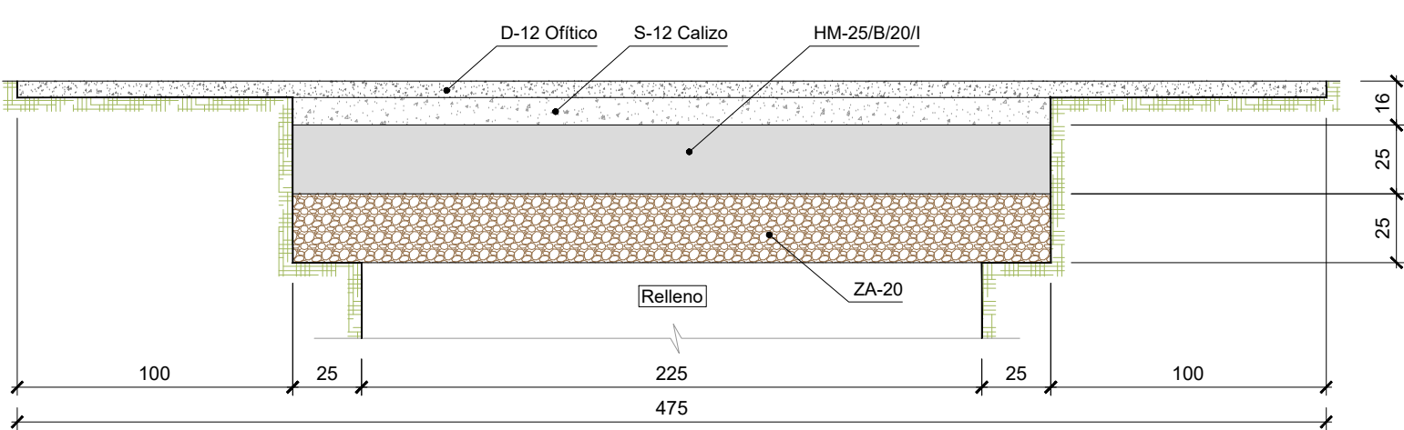
SECCIÓN TIPO PAQUETE DE REPOSICIÓN DE PAVIMENTO ASFÁLTICO EN ZANJA. E=1/25
