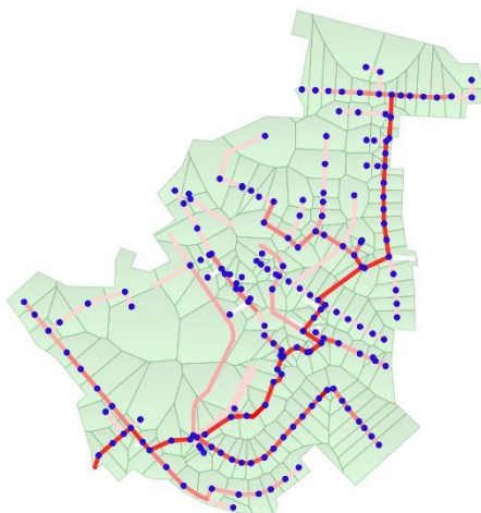
Esquema de cuencas discretizadas en el modelo
