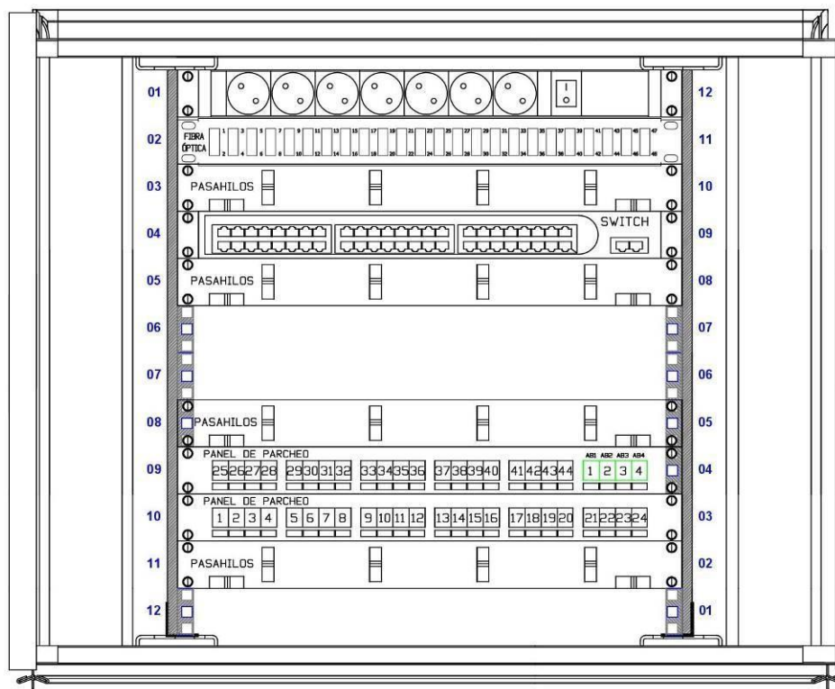
Esquema ejemplo de armario concentrador de 12U:
