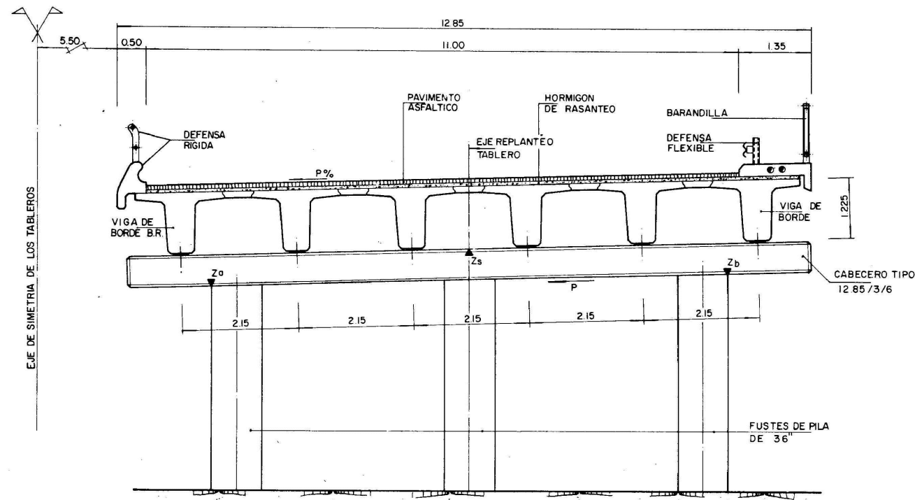
SECCION TRANSVERSAL TIPO ESCALA 1:50
