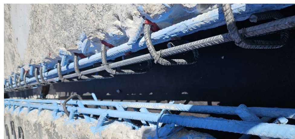
RECONSTRUCCIÓN DE BORDES DE TABLERO
