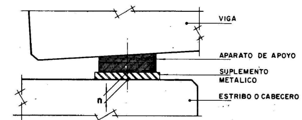
ESQUEMA DE APARATO DE APOYO (SECCION POR EJE DE VIGA)
