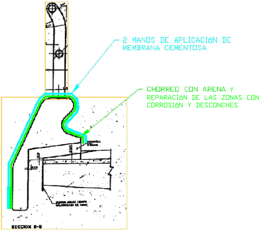
DETALLE IMPOSTA CARRIL IZQUIERDO
