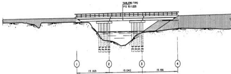
ALZADO (CALZADA DERECHA) ESCALA 1:250
