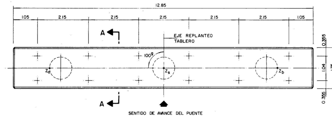
SITUACION EJES APARATOS DE APOYO EN CABECEROS ESCALA 1:50
