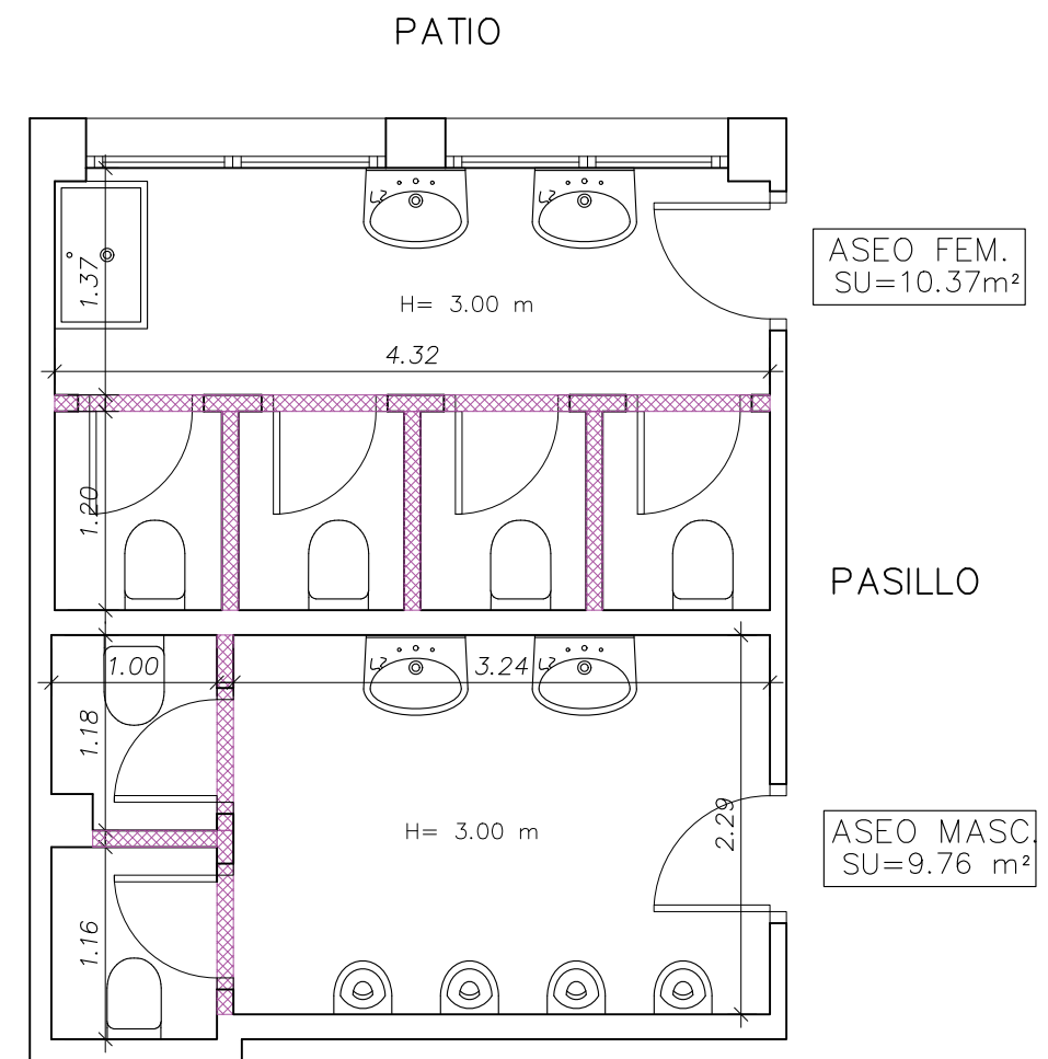
PLANTA SEGUNDA
