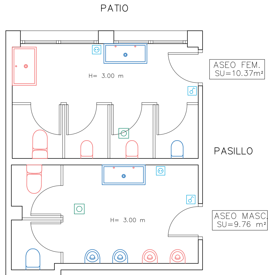
PLANTA PRIMERA
