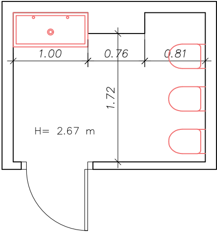
BAÑO INFANTIL 1
