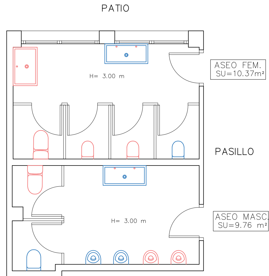
PLANTA PRIMERA
