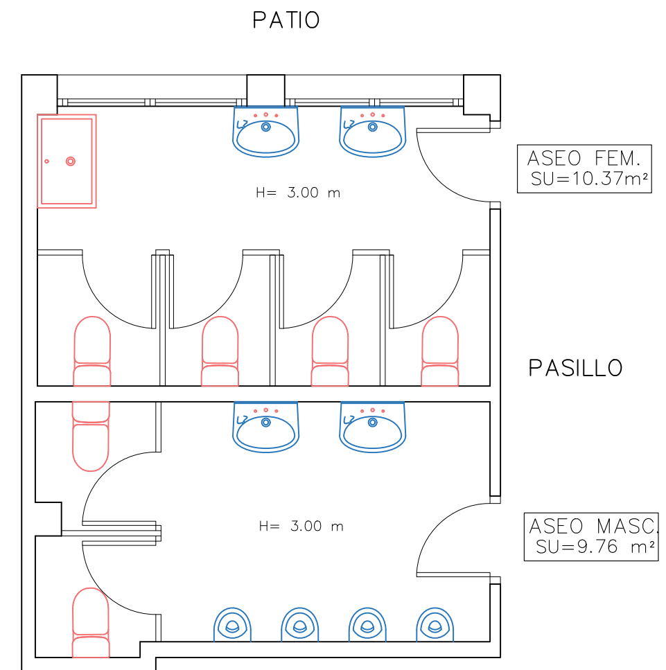
PLANTA SEGUNDA
