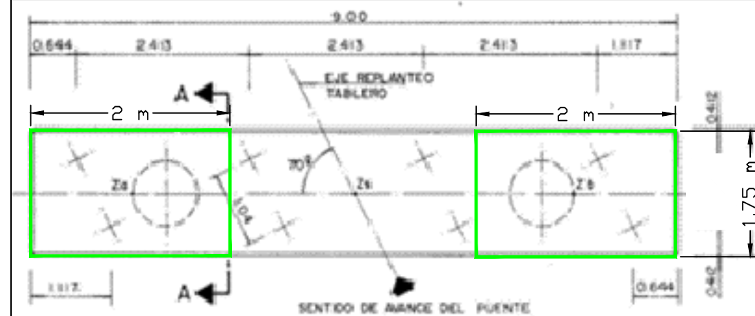
SITUACION EJES APARATOS DE APOYO EN CABECEROS
