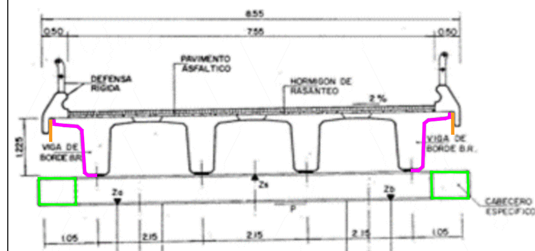
SECCIÓN TRANSVERSAL TABLERO
