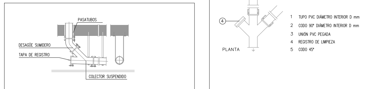
DETALLE DE SANEAMIENTO COLGADO (PLANTA)
