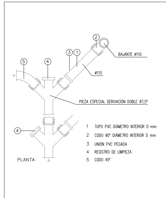
DETALLE DE SANEAMIENTO COLGADO (PLANTA)
