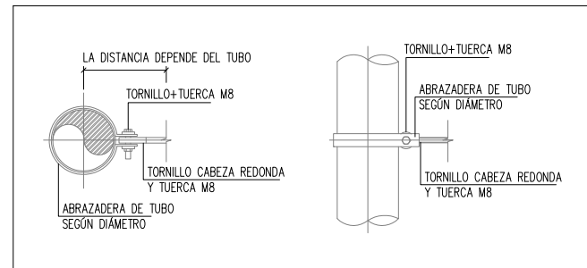
DETALLE DE SANEAMIENTO COLGADO
