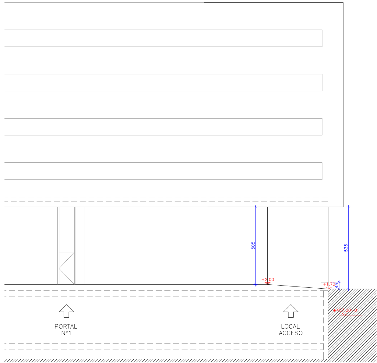
ALZADO NORTE
