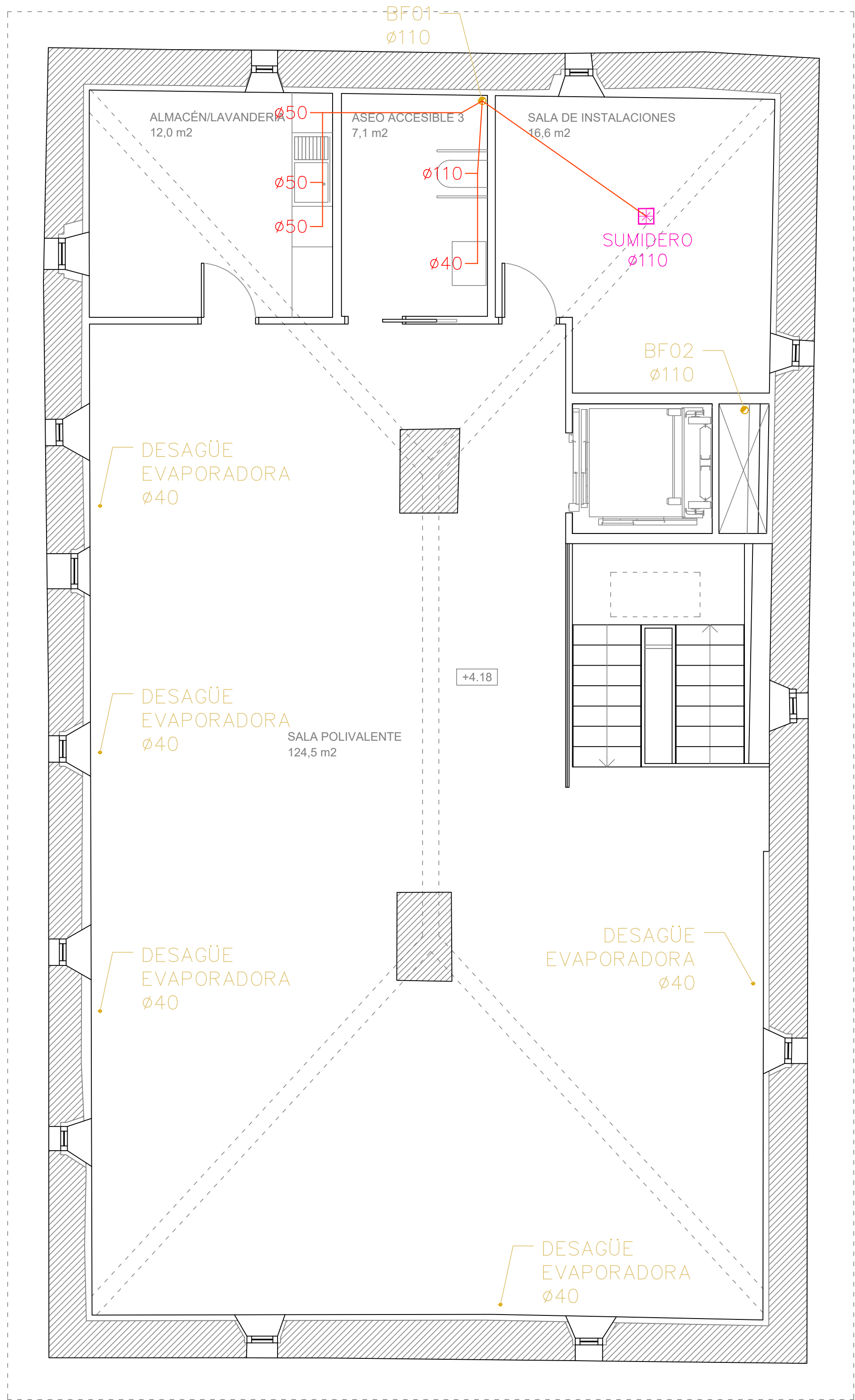
PL. BAJOCUBIERTA
