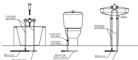
BAÑO DETALLE ACOMETIDAS A APARATOS SANITARIOS
