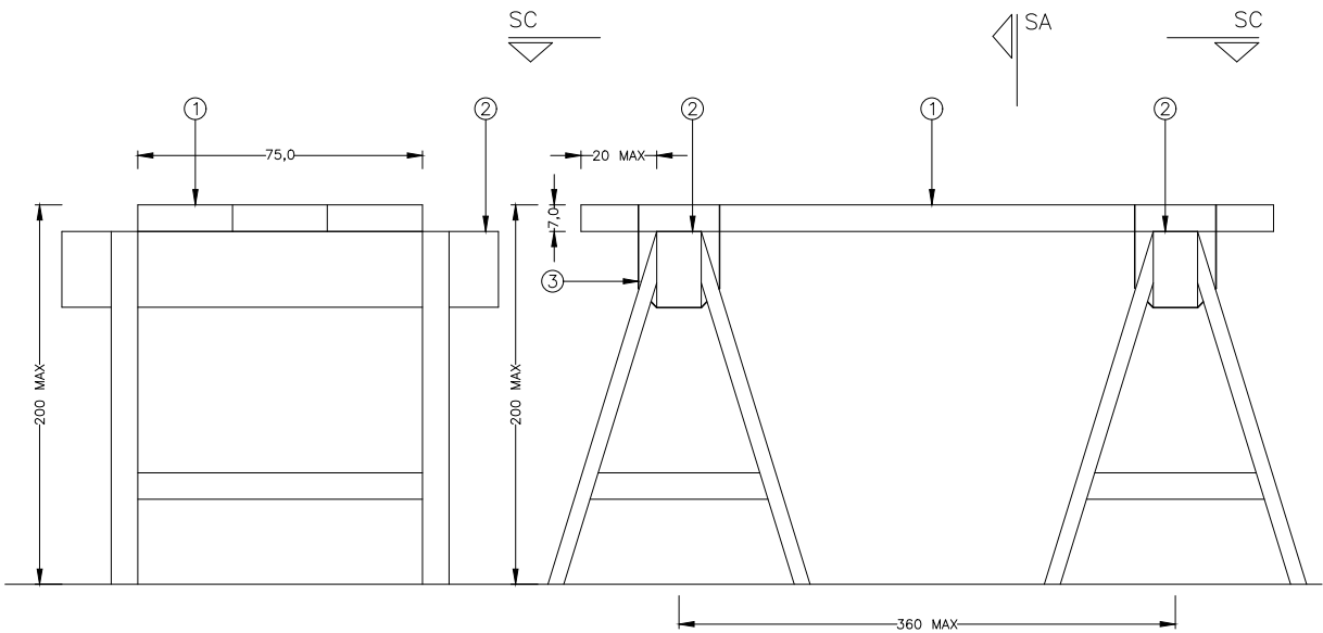
SECCIÓN A-A
