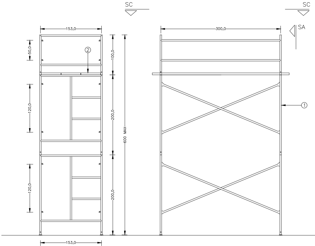
SECCIÓN A-A
