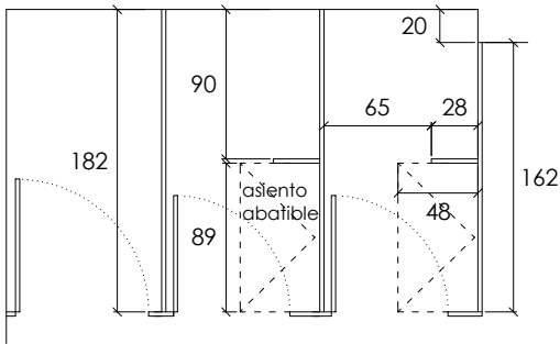
C3 Mampara sanitaria de tablero fenólico 25 mm 3 puertas abatibles + 2 asientos abatibles
