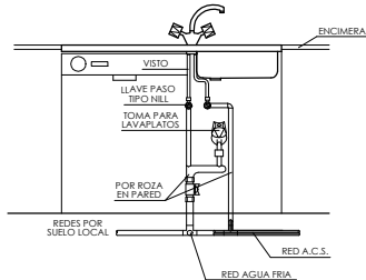
COCINA DETALLE ACOMETIDA A APARATOS SANITARIOS
