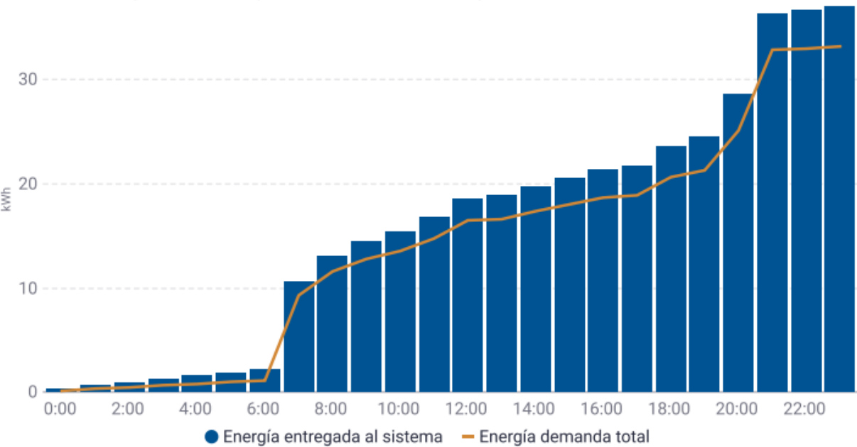
Demanda vs producción (día más desfavorable)
