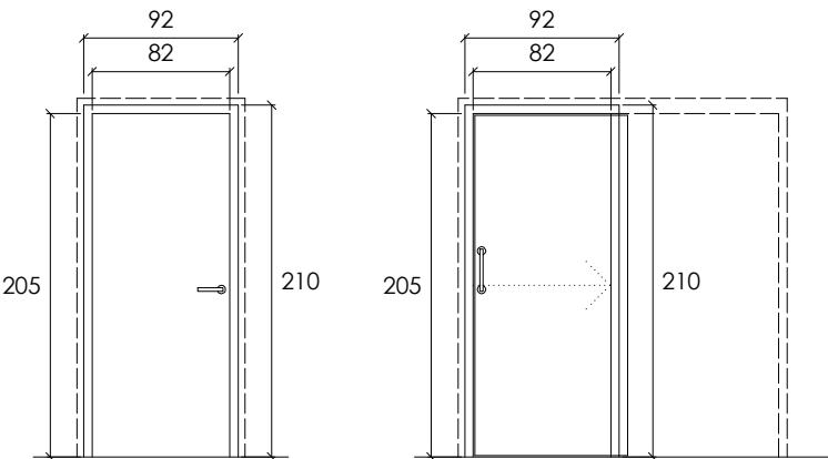
C1 Puerta interior de DM - lacada abatible C2 Doble Puerta interior de DM - lacada corredera
