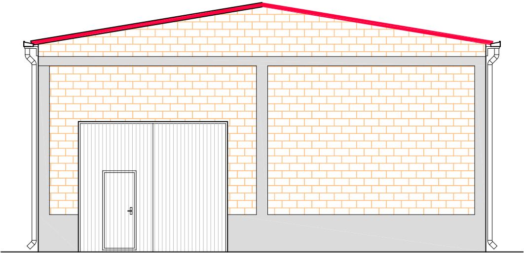
ALZADO SUR
