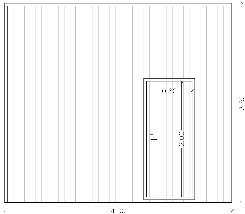
PUERTA ABATIBLE DE CHAPA TIPO PEGASO ACABADA EN COLOR ROJO CON PUERTA PEATONAL INCRUSTADA 2 UNIDADES
