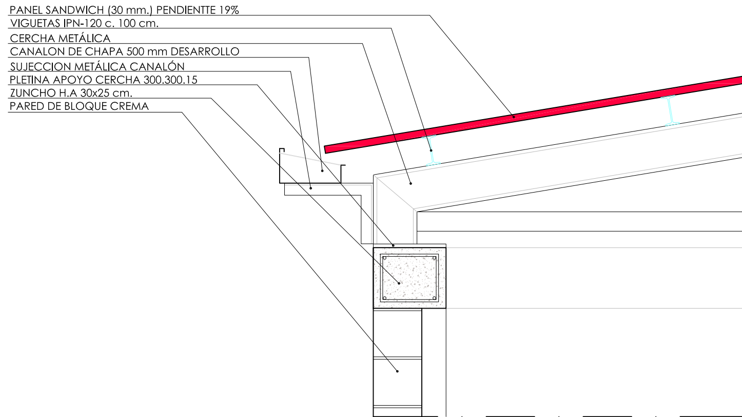
DETALLE ALERO (E:1:20)
