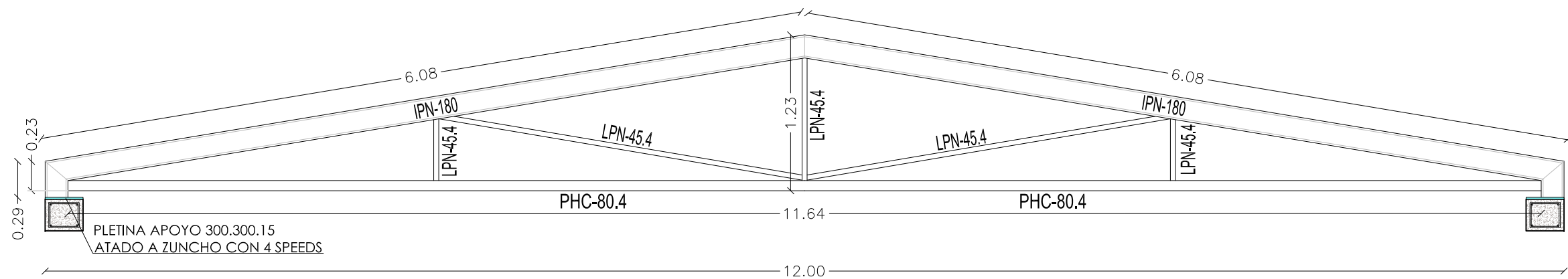
DETALLE CERCHA (E:1:40)
