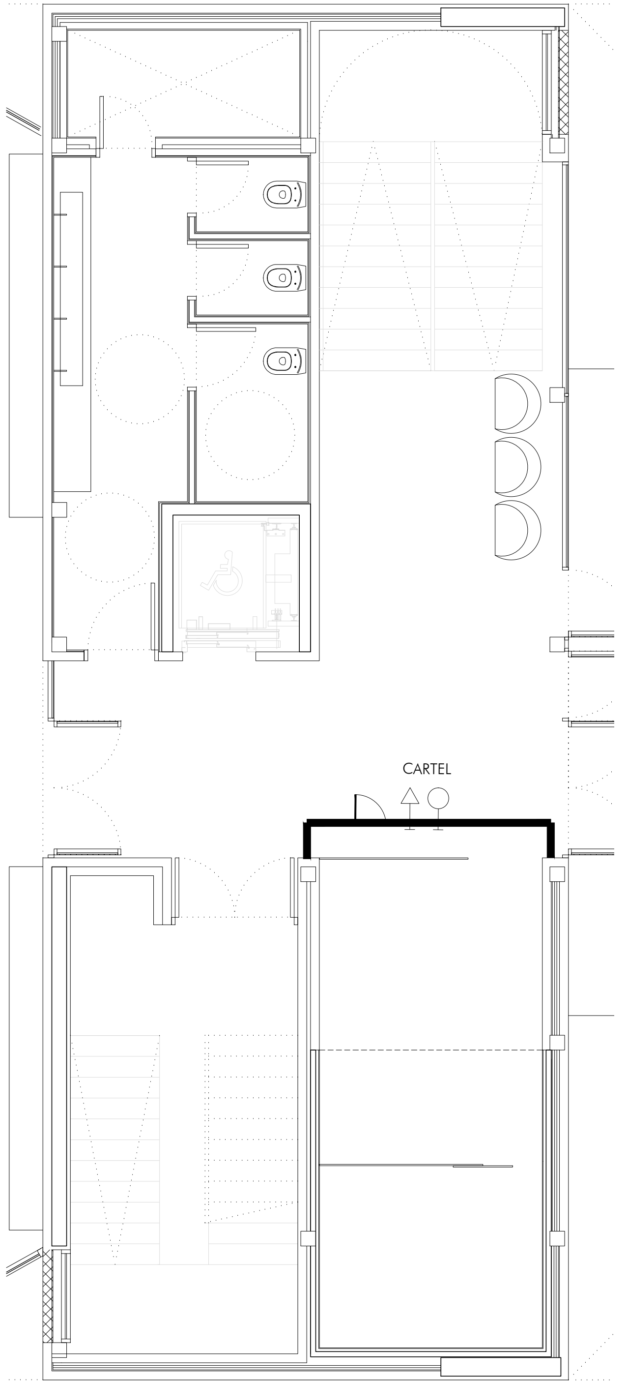
PLANTA BAJA
