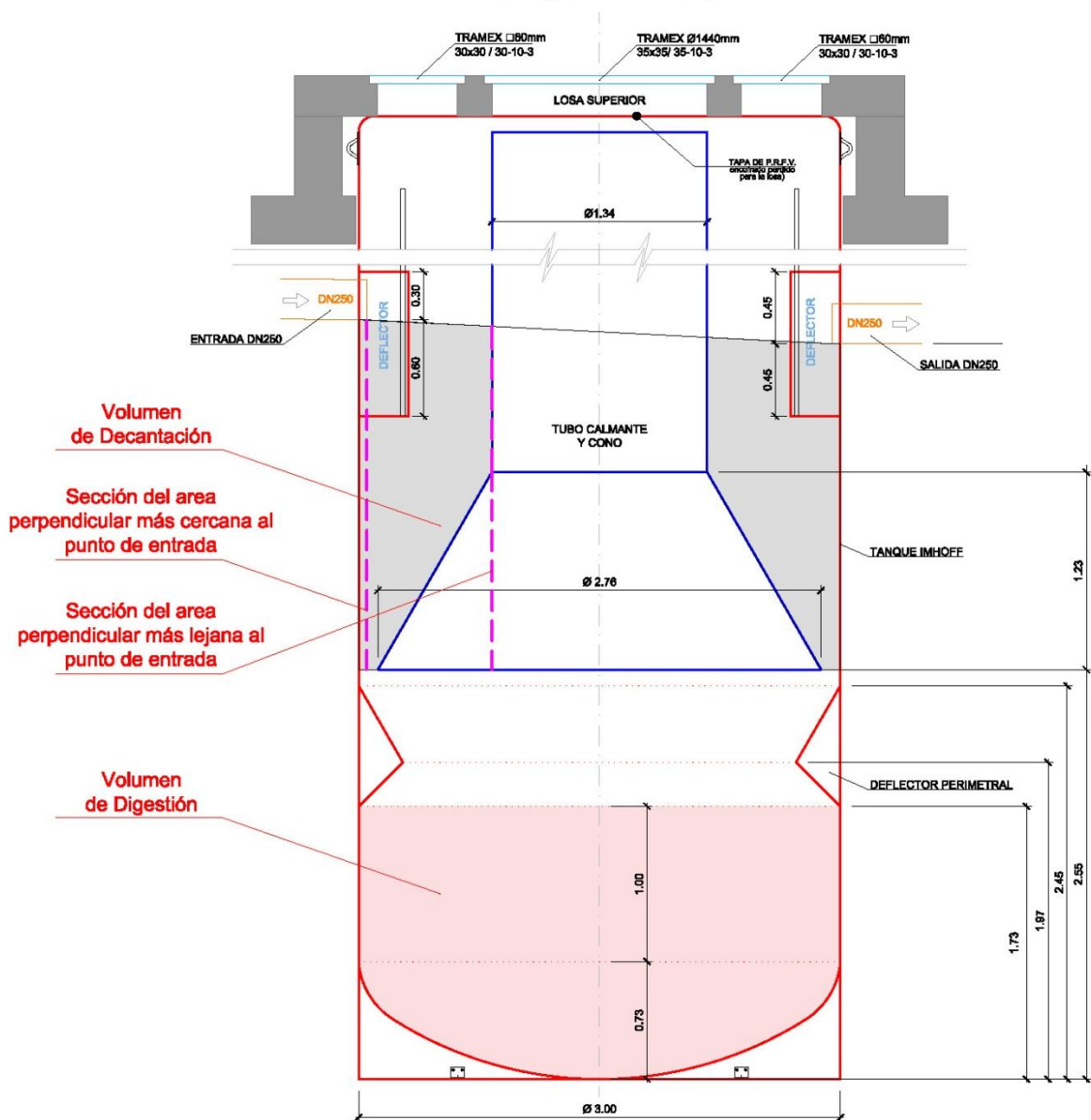
IMHOFF (Sección/Alzado)
