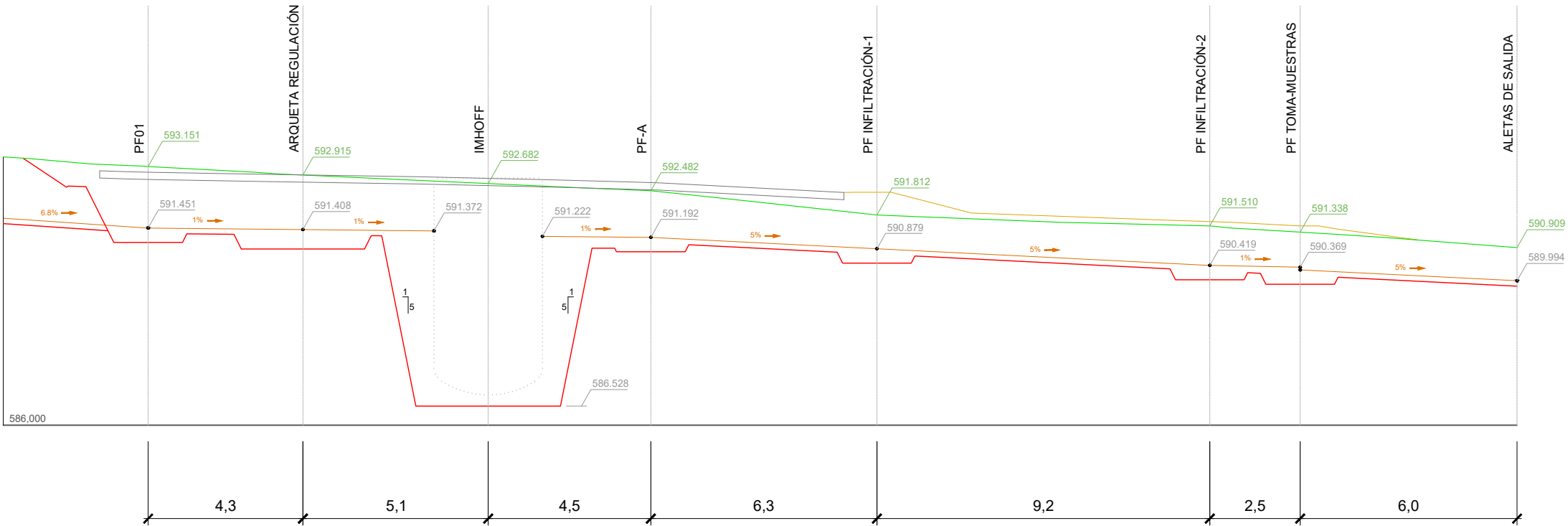
PERFIL DE LÍNEA DE AGUA SIMPLIFICADO
