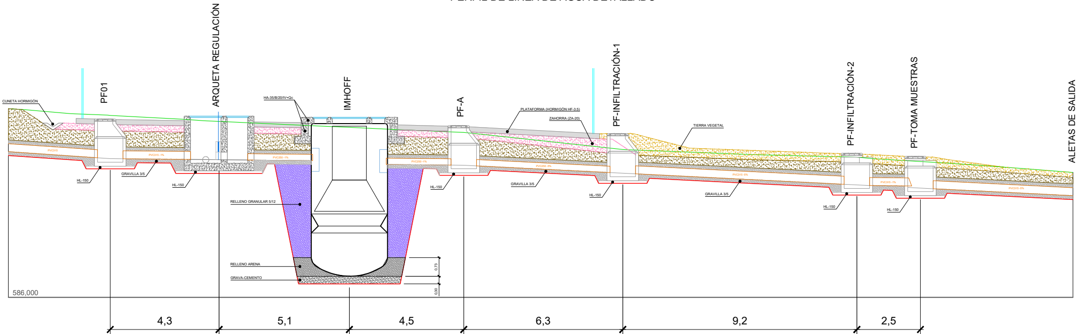
PERFIL DE LÍNEA DE AGUA DETALLADO
