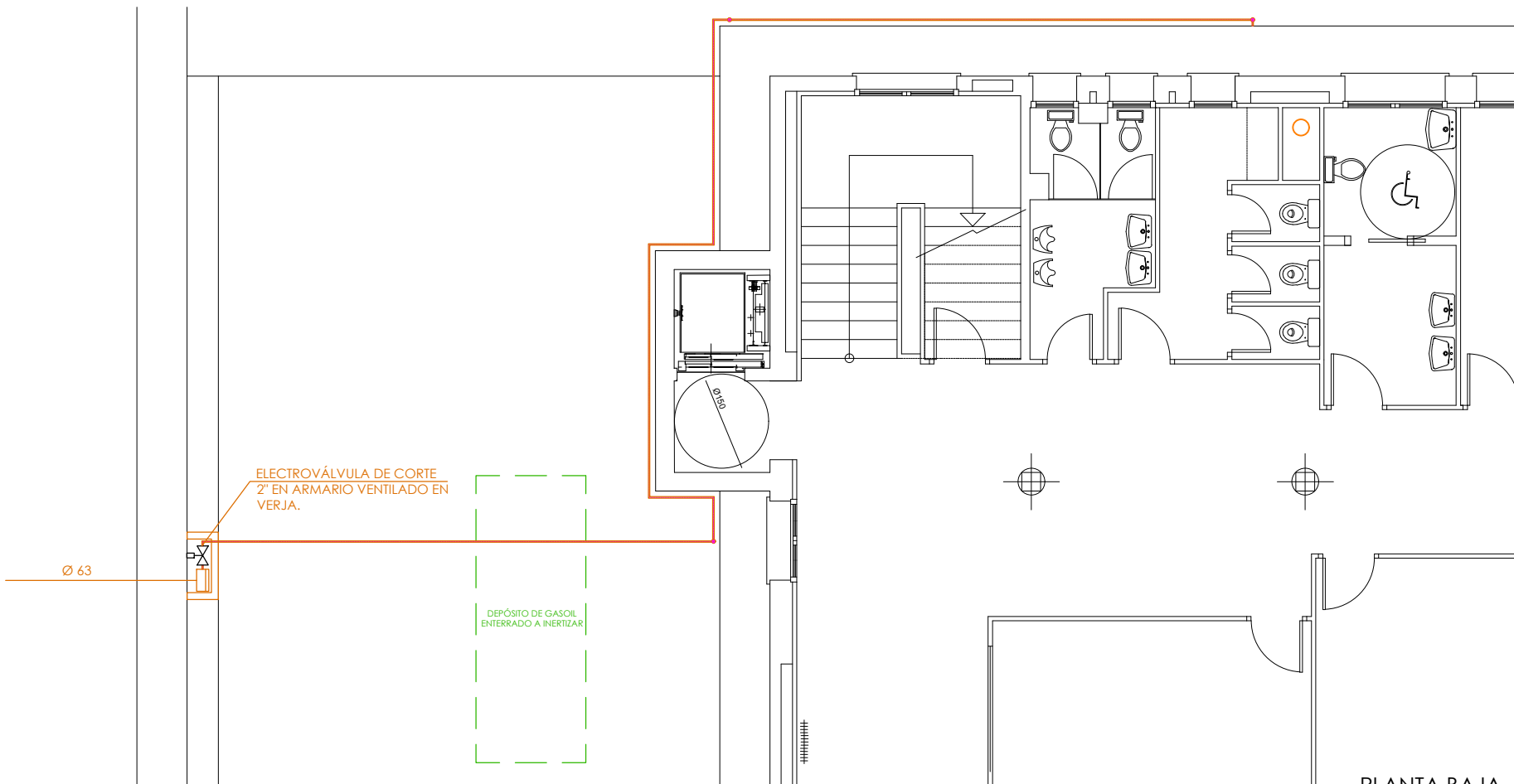
PLANTA BAJA
