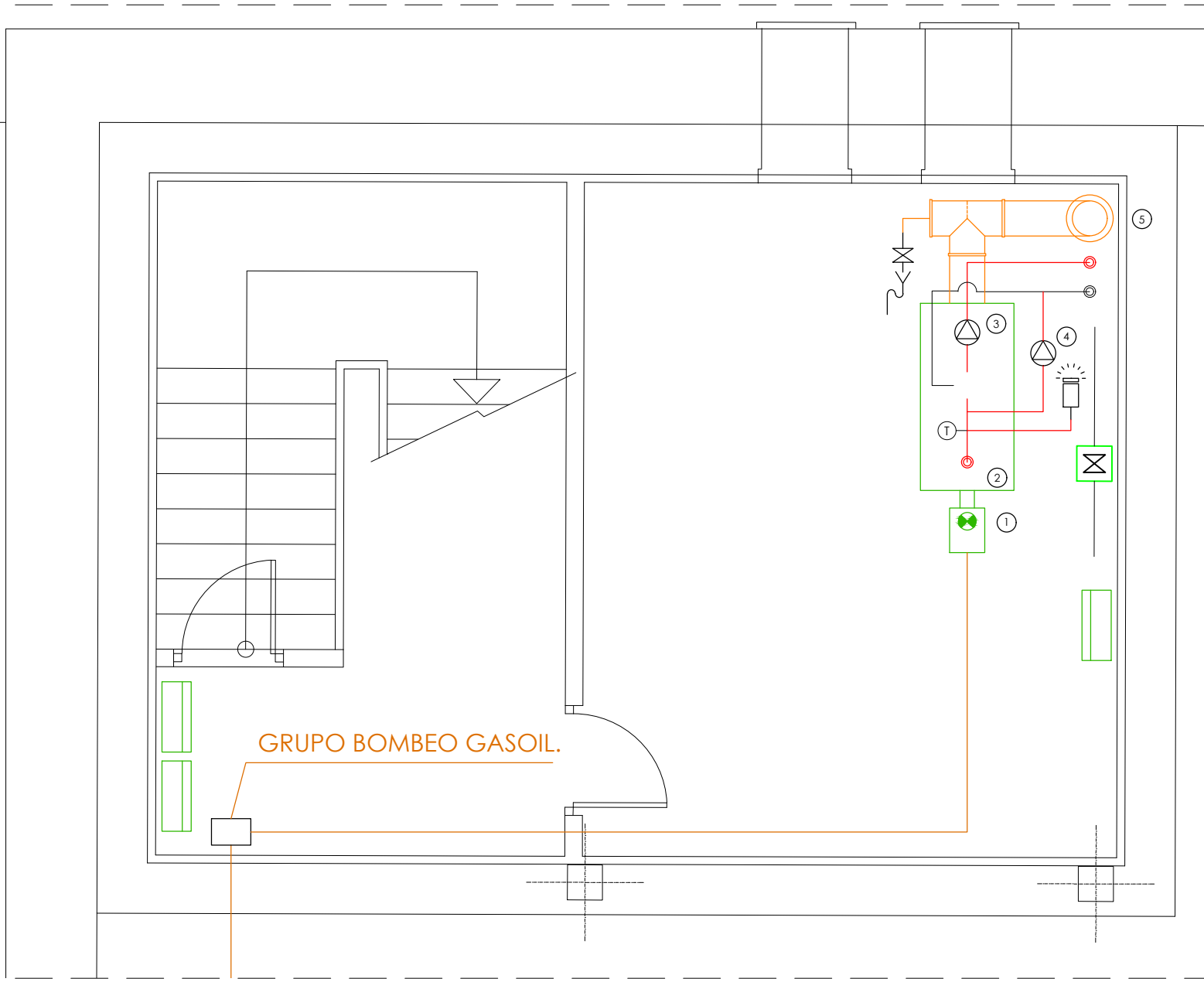
PLANTA SÓTANO -1
