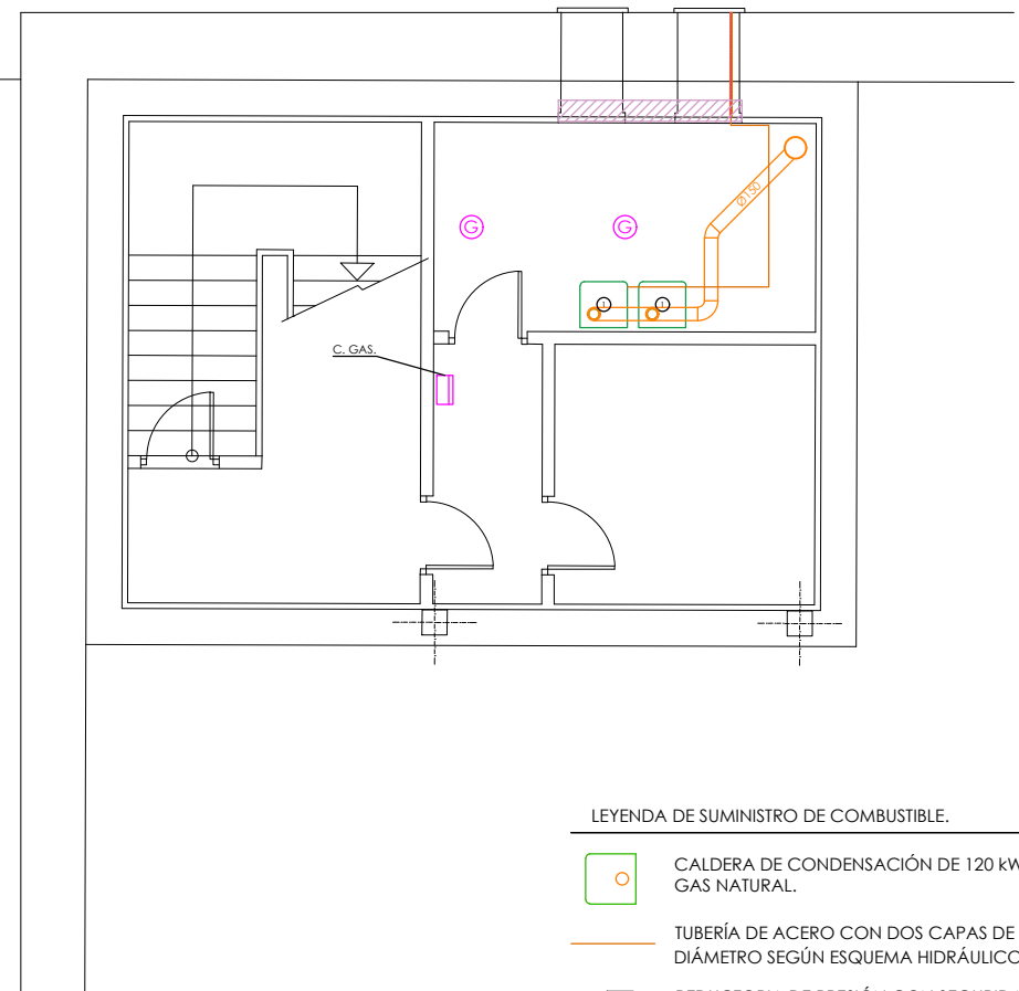
PLANTA SÓTANO -1
