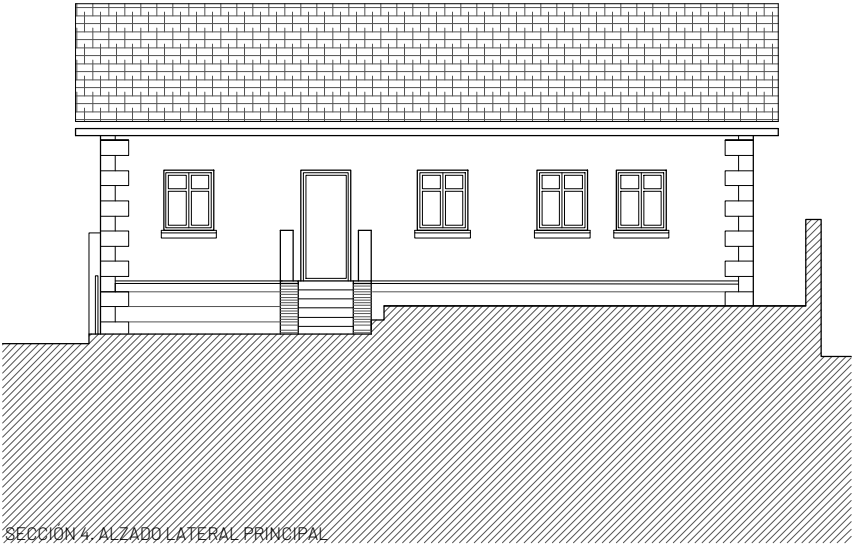
SECCION 4. ALZADO LATERAL PRINCIPAL
