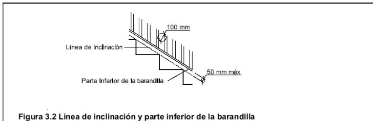
Figura 3.2 Línea de inclinación y parte inferior de la barandilla
