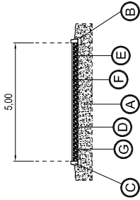
PERFIL ZONA PETANCA
