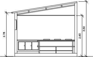
SECCION A-B
