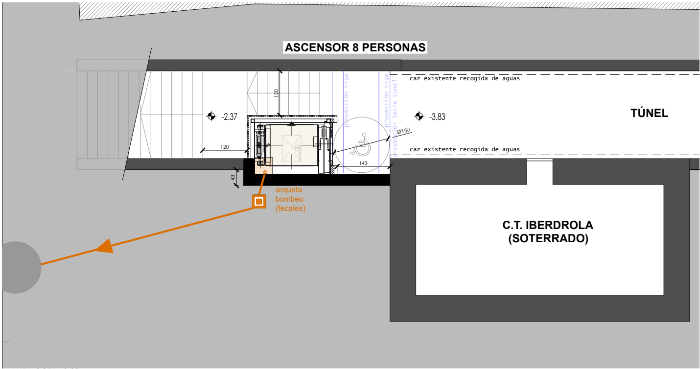
PLANTA COTA -3.83
