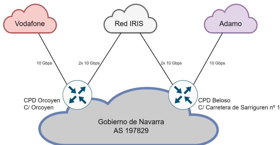
Figura 1: Esquema actual de tránsitos a Internet de GN
