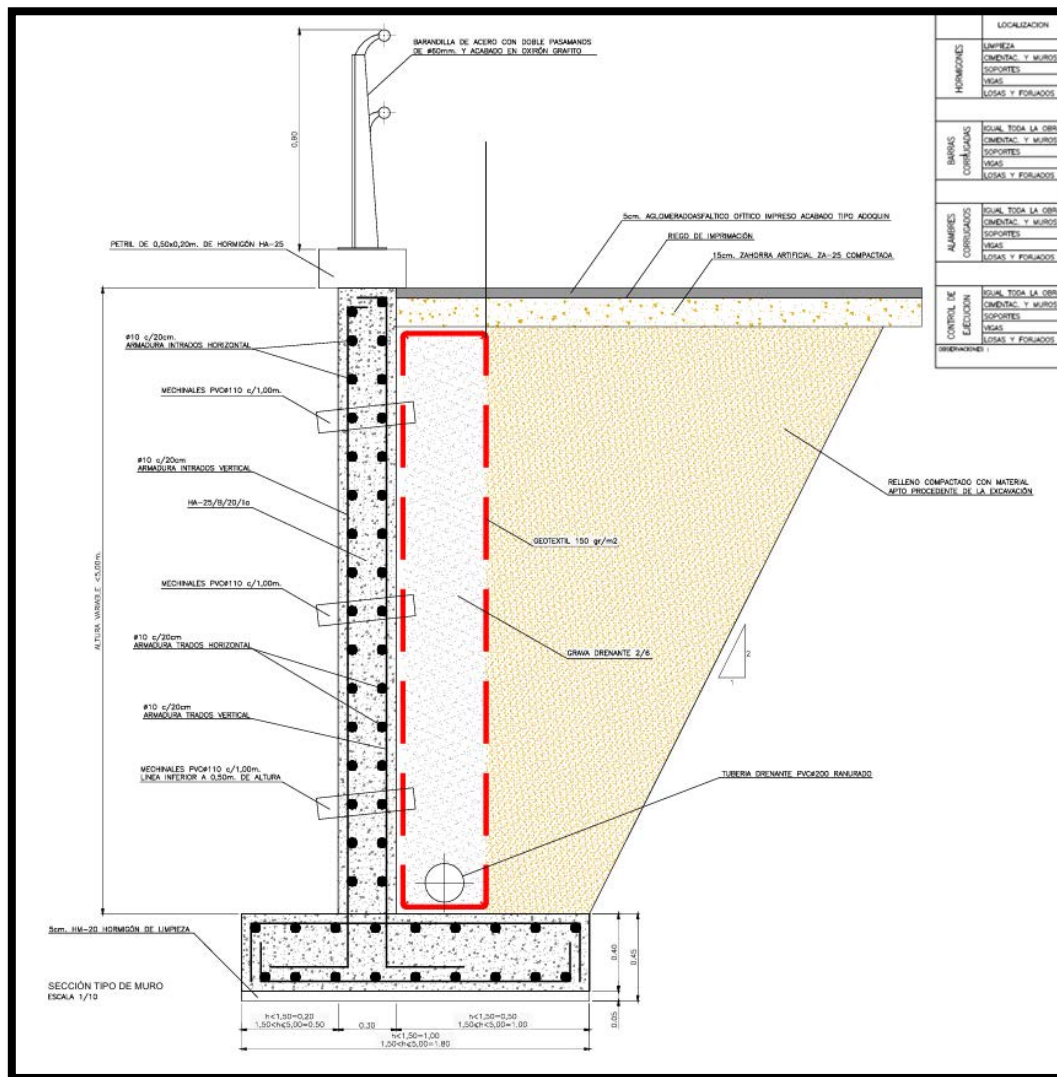
Imagen 17: Ventana del plano del muro y sus detalles de armado
