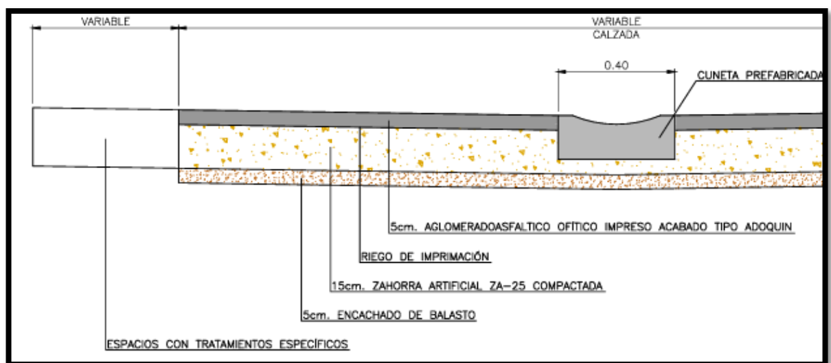
Detalle del firme
