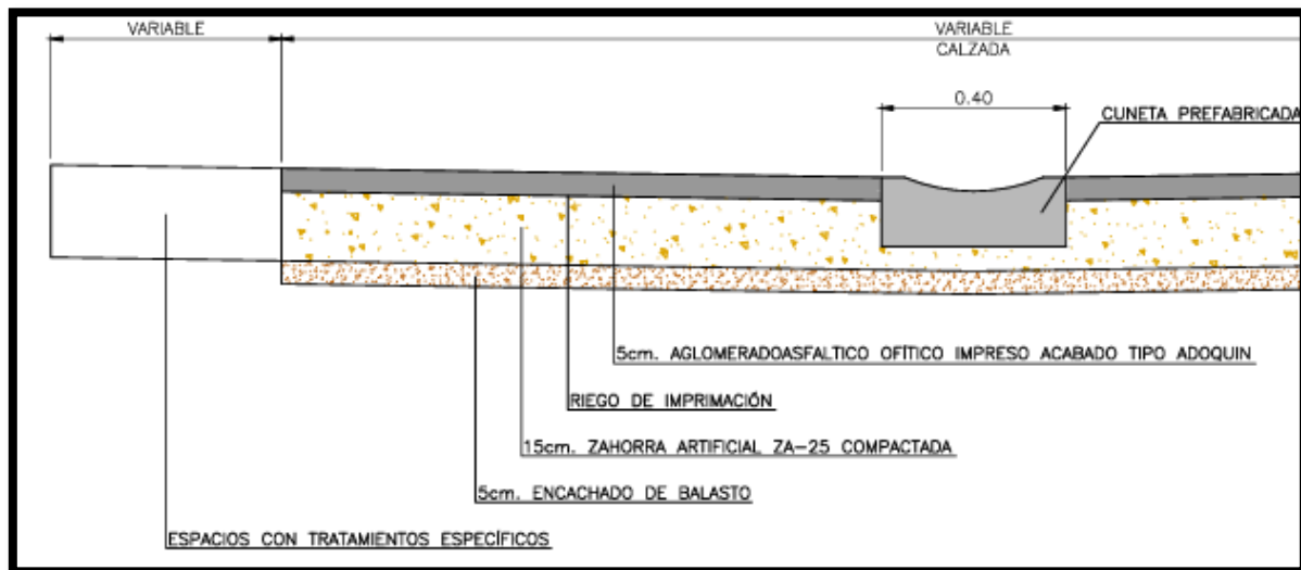
Imagen 18: Detalle del firme
