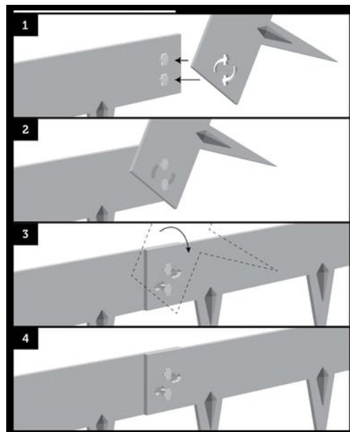
Imagen 21y 22: Foto y detalles constructivos de bordura Multi-Edge METAL Galvanizado
