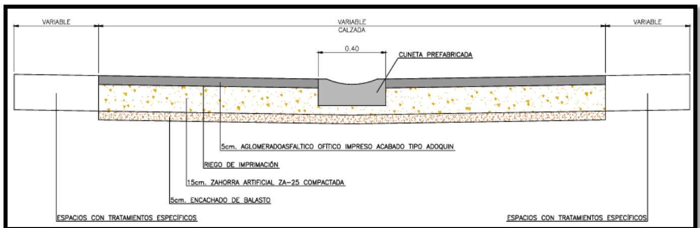
Imagen 4: Sección de la solución proyectada.
