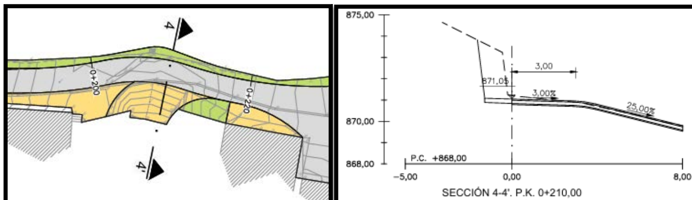
Imágenes 14 y 15: Actuación en punto singular “vieira”
