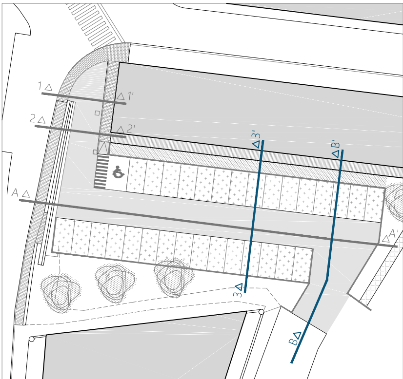
PLANTA ACTUACION E 1/500
