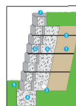
MURO REFORZADO CON GEORED GEOGRID WALL SECTION
