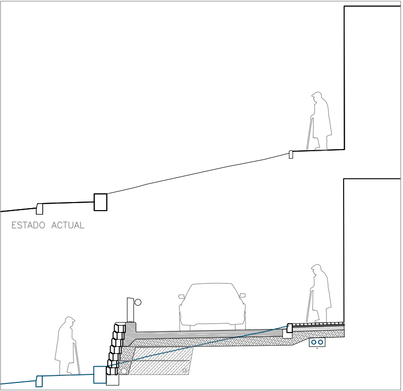
PROPUESTA SECCIÓN 2-2' E 1/100
