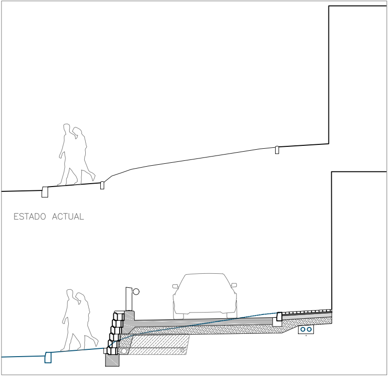
PROPUESTA SECCIÓN 1-1' E 1/100
