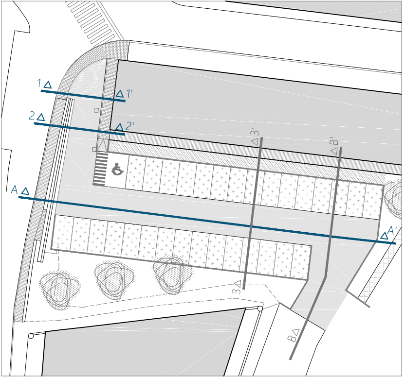
PLANTA ACTUACION E 1/500
