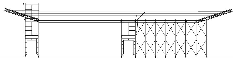
VISERA PROTECCION
