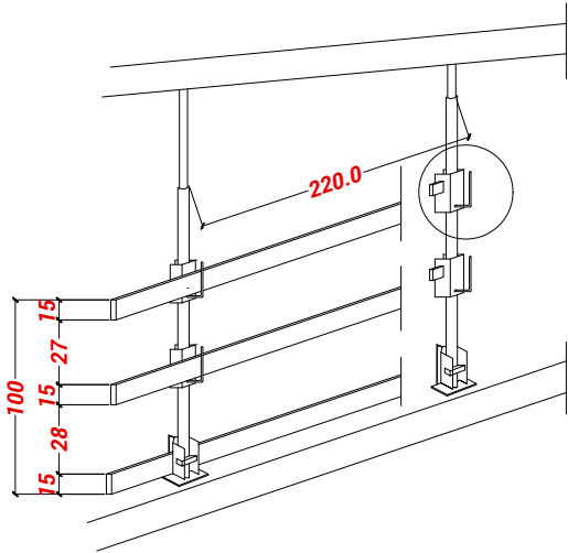
BARANDILLAS FORJADOS .
