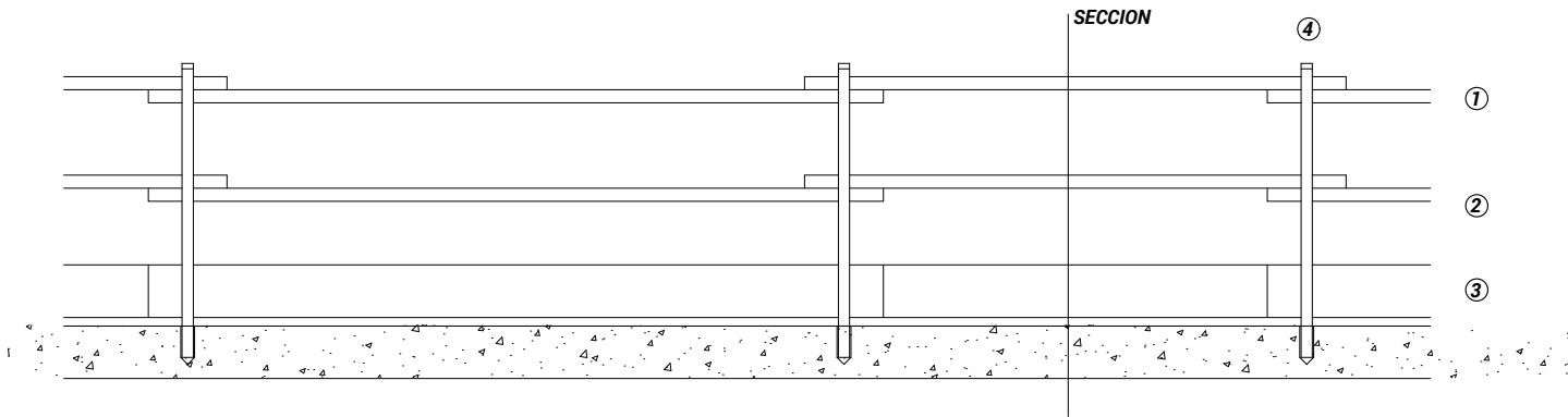
ALZADO
