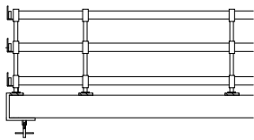
BARANDILLAS ALERO
