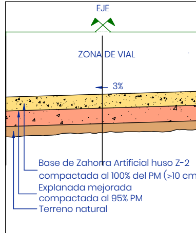
SECCIÓN TIPO CAMINO EN TIERRAS ESCALA: S/E
