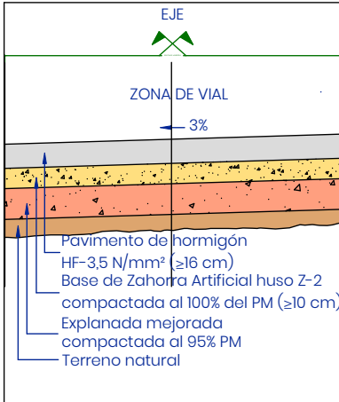
SECCIÓN TIPO PAVIMENTO DE HORMIGÓN ESCALA: S/E
