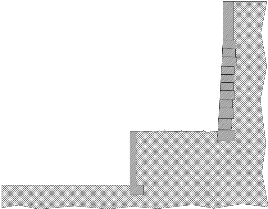
ESTADO ACTUAL SECCION TRANSVERSAL MURO, ESCALA 1/75
