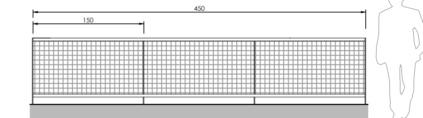
BARANDILLA B1 (sobre muro)
