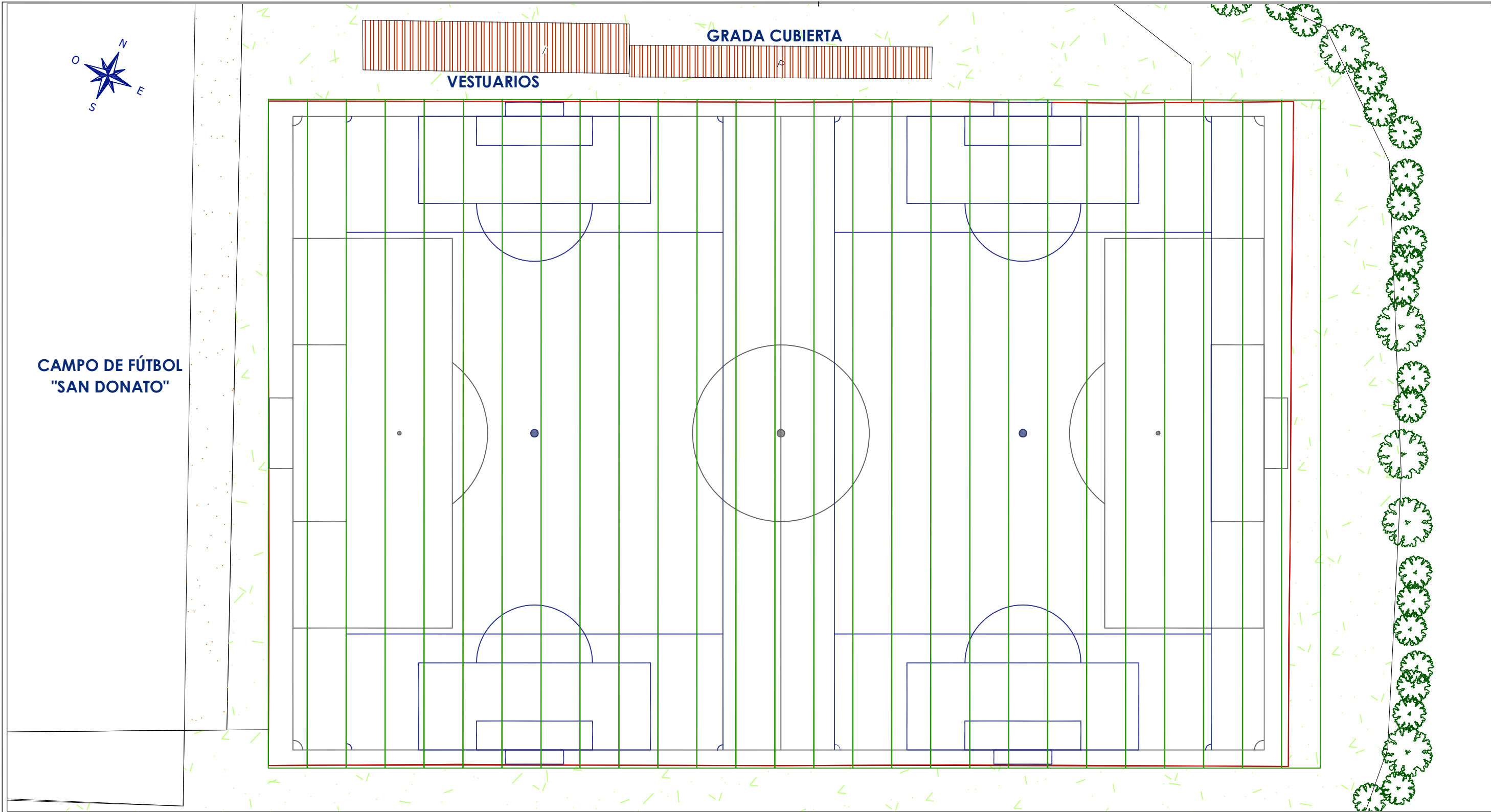
DETALLE ENCOLADO DE JUNTAS Y LINEAS DE JUEGO
