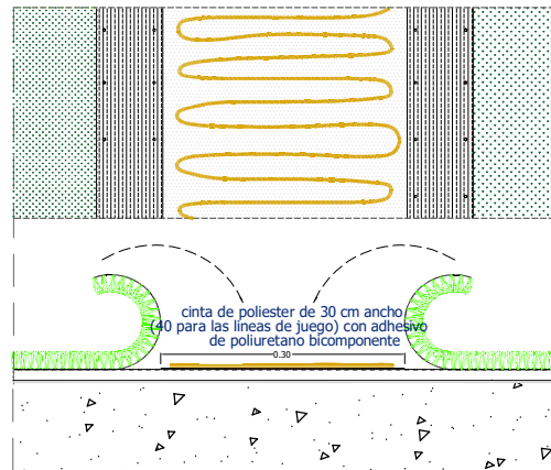
DETALLE ENCOLADO DE JUNTAS Y LINEAS DE JUEGO
