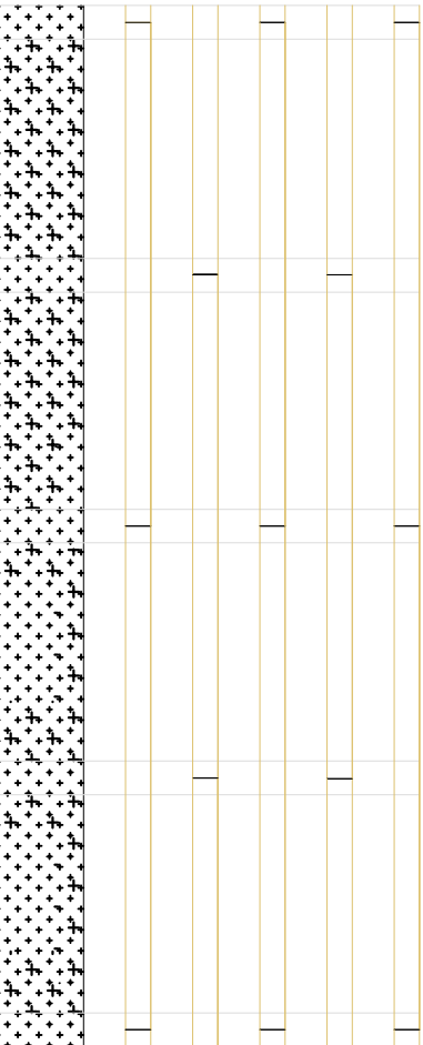
Detalle colocación largueros al tresbolillo
