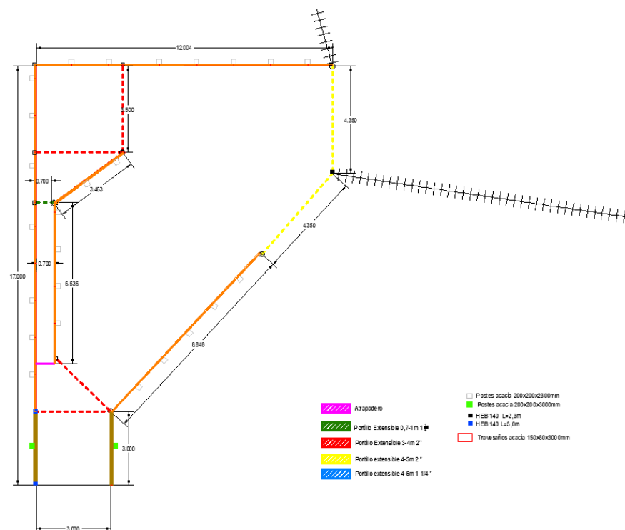
Imagen nº5: Planta manga, Trazado color rojo zona cerrada con postes de madera. En trazo discontinuos portillos: Amarillo longitud 4-5 m, verde longitud 0,7 m y rojo longitud 3-4 m
