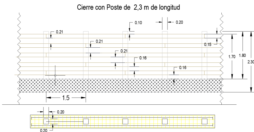
Imagen nº6: Perfil transversal del cierre de la manga
