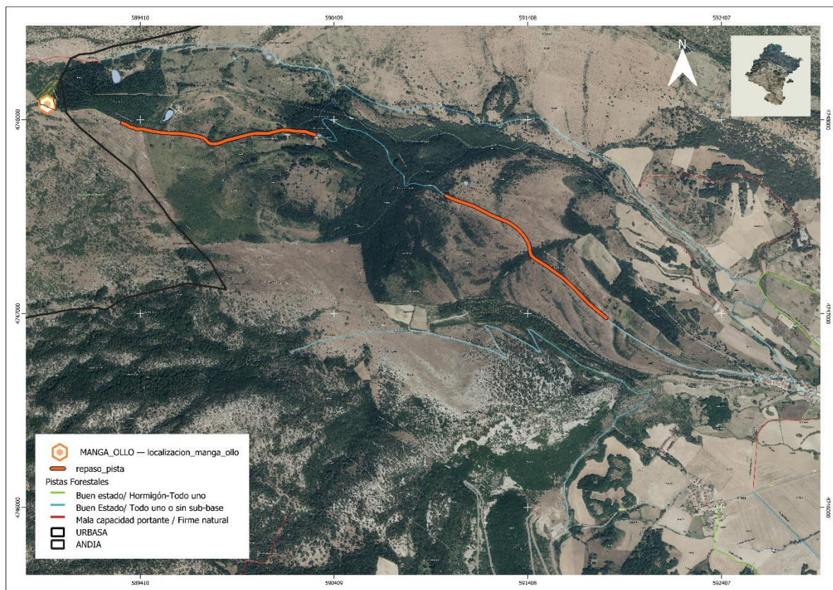
Imagen nº14: Tramos a realizar repaso pistas y cunetas.
