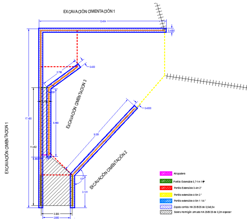
Imagen4: Planta manga, Rayado de azul excavación de zanja corrida de 50x60 cm a hormigonera una vez los postes se hayan presentado.
