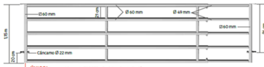
Imagen nº10: Perfil transversal portillos extensibles de 3-4 y 4-5 metros de anchura y 2" de espesor
