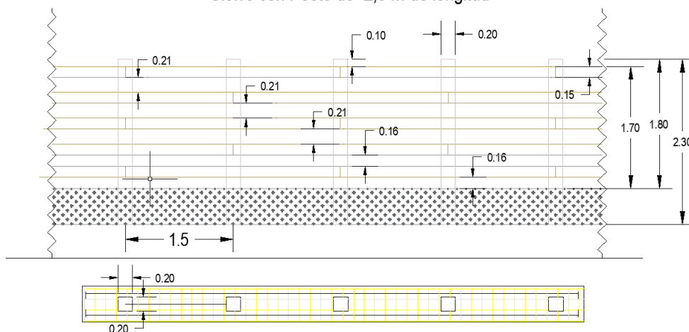
Cierre con Poste de 2,3 m de longitud
