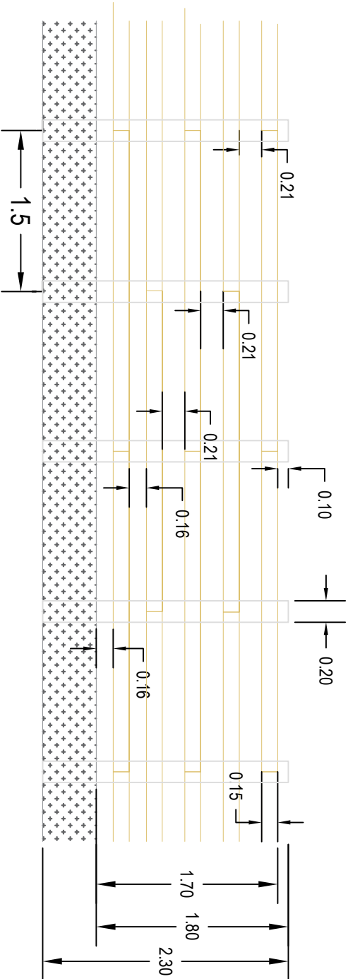
Cierre con Poste de 2,3 m de longitud
