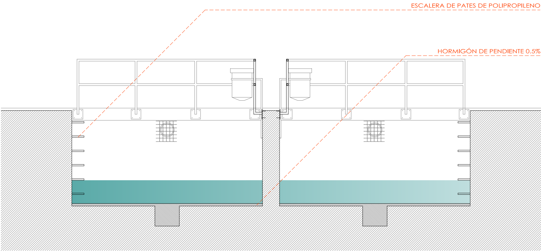
SECCIÓN TANQUE TRANSVERSAL. ESTADO REFORMADO
