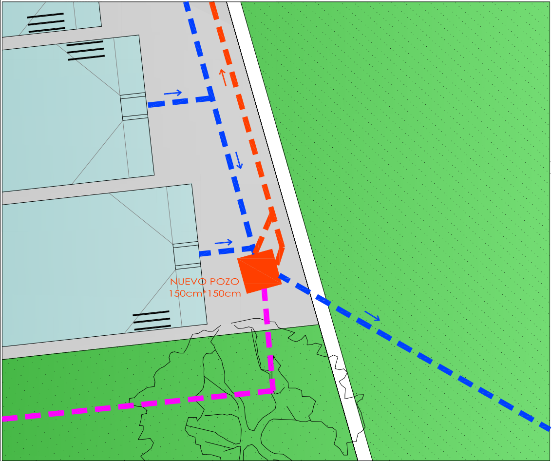
ESTADO REFORMADO
