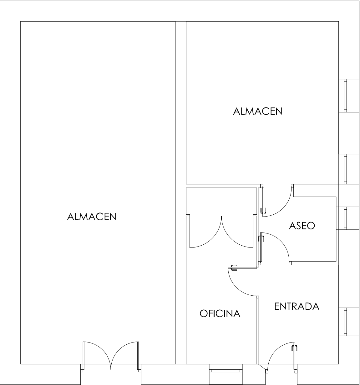
ESTADO ACTUAL
