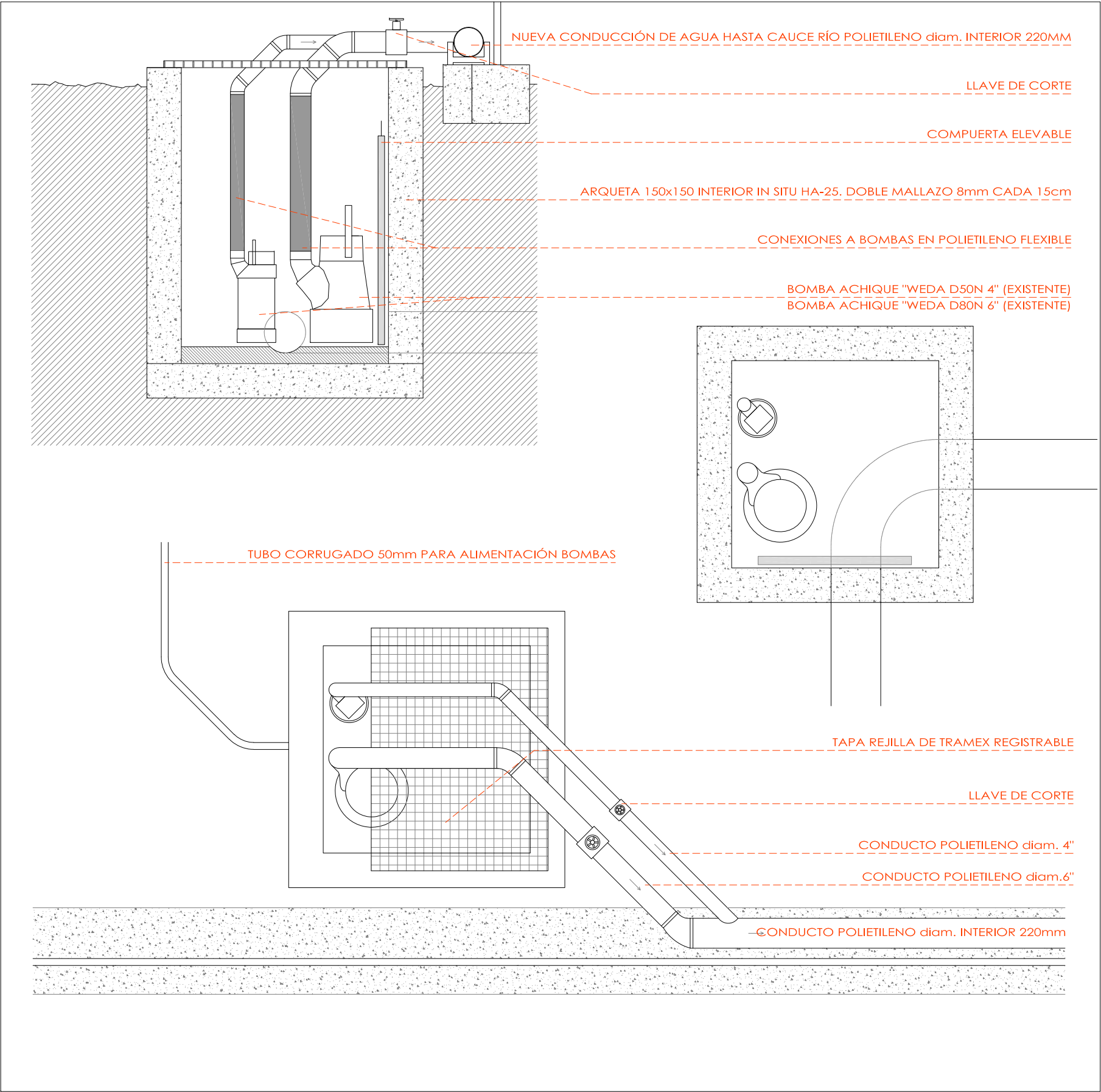
DETALLE NUEVO POZO BOMBAS
