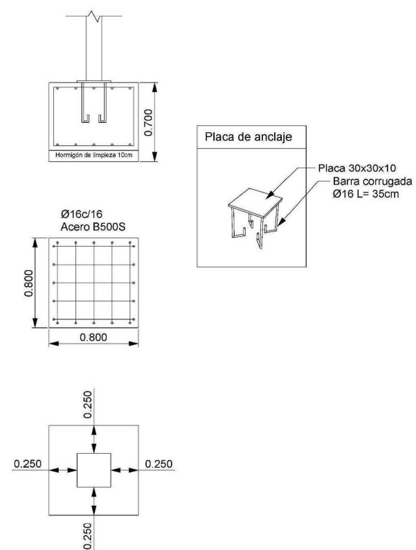
Zapata Z1: 5 Uds
