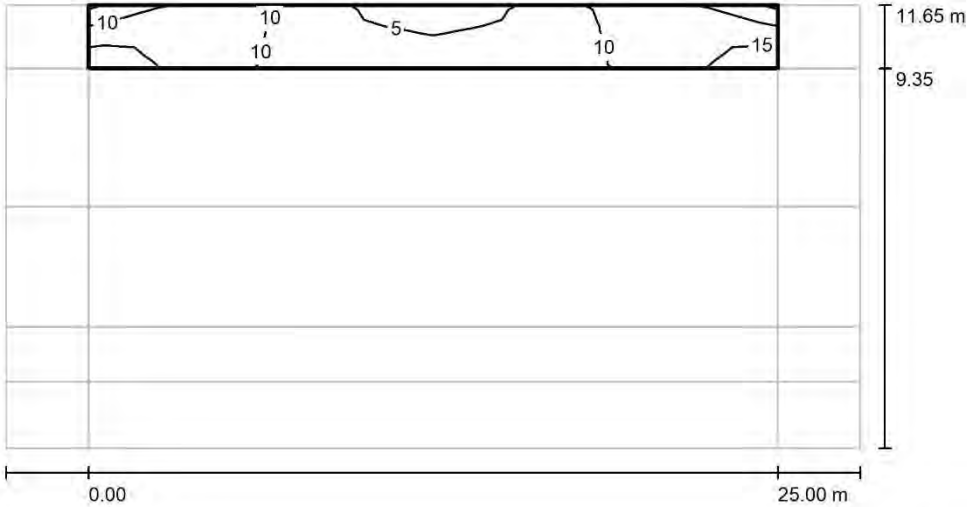
Sección (unilateral) / Recuadro de evaluación Camino peatonal 1 / Isolíneas (E)
