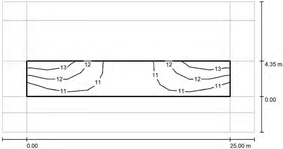
Sección (unilateral) / Recuadro de evaluación Calzada 1 / Isolíneas (E)
