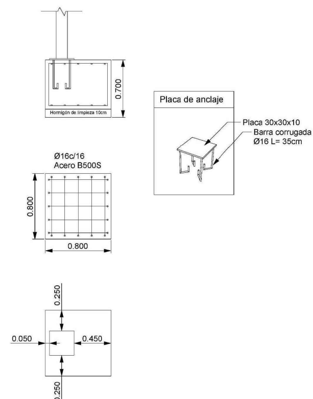
Zapata Z2: 3 Uds
