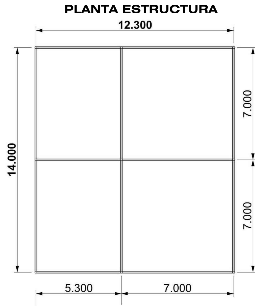
Zapata Z1: 5 Uds
