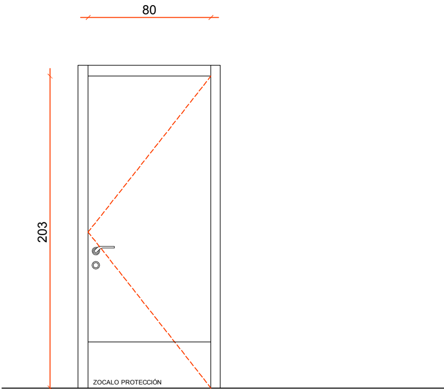
P.1 4 UNIDADES CON CONDENA
