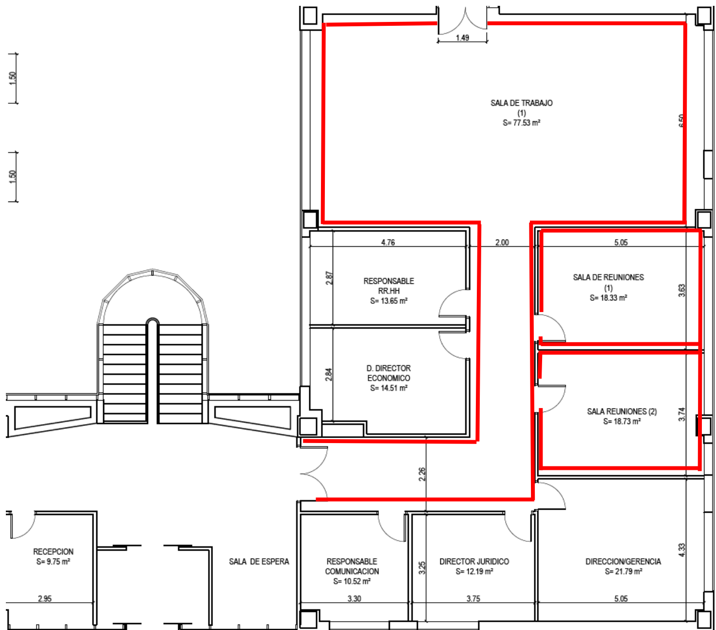
PLANTA BAJA
