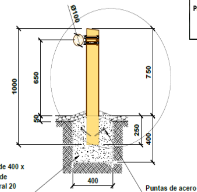
SECCIÓN DADA POR EJE DE POSTE
