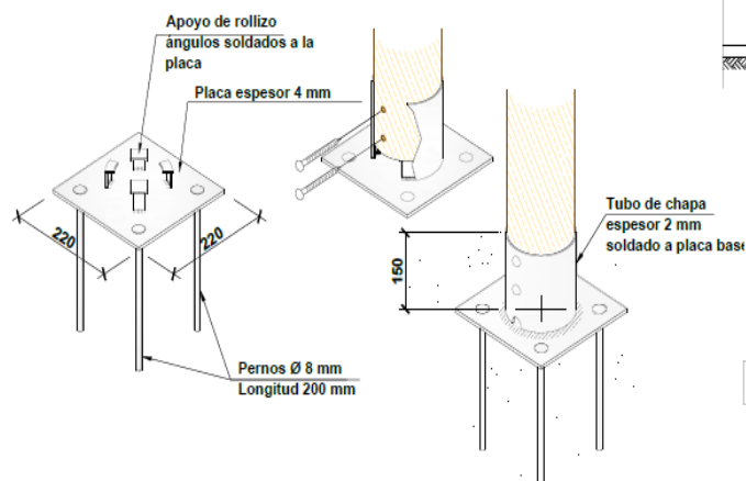
ANCLAJE EN ROCA U HORMIGÓN EXISTENTE
