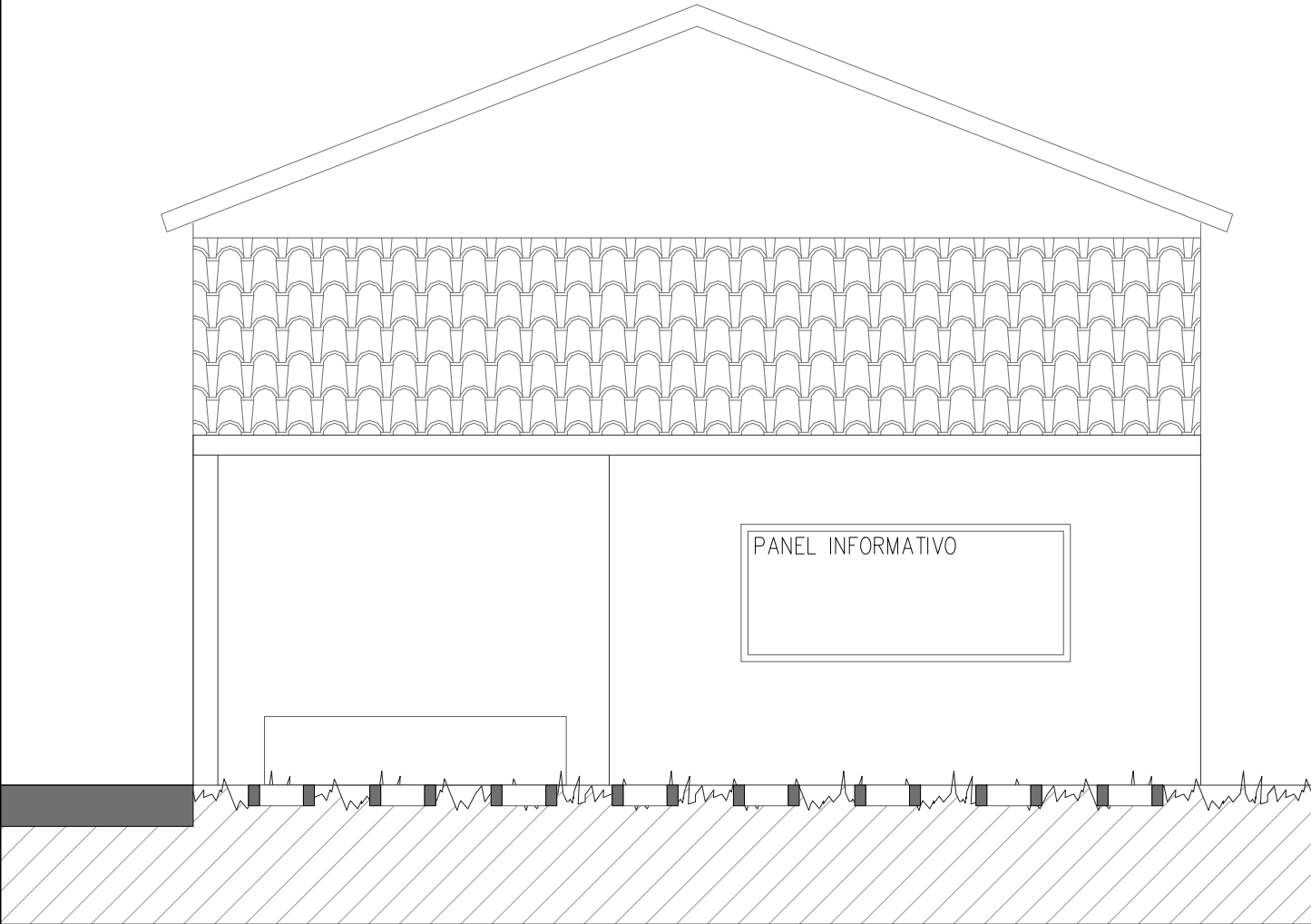
SECCIÓN A-A' E:1:50
